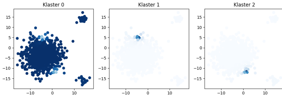
Rysunek 5.23: Przynależność punktów do klastrów dla danych ‘blobs’ o rozmiarze 1000.
