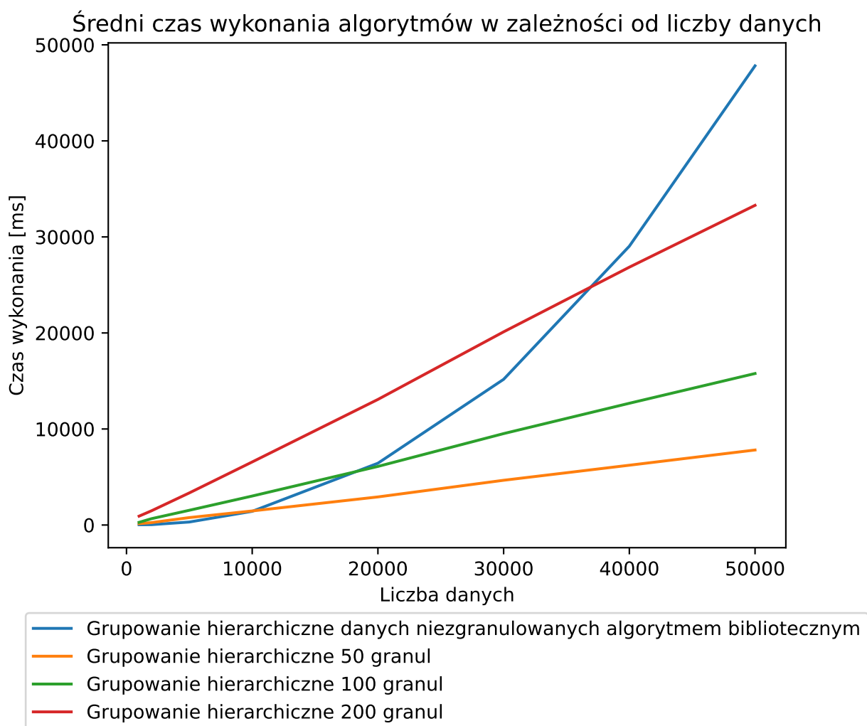
Rysunek 5.7: Charakterystyka czasu wykonania algorytmu ostrego AgglomerativeClustering biblioteki scikit-learn i własnej implementacji algorytmu rozmytego dla różnej liczby granul od liczby danych wejściowych.
