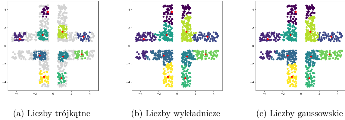
Rysunek 5.5: Przynależność punktów do granul w zależności od kształtu liczb rozmytych. 10 środków granul oznaczono kolorem czerwonym, punkty należące do różnych granul oznaczone są różnymi kolorami. Kolorem szarym oznaczono punkty stanowiące szum.
