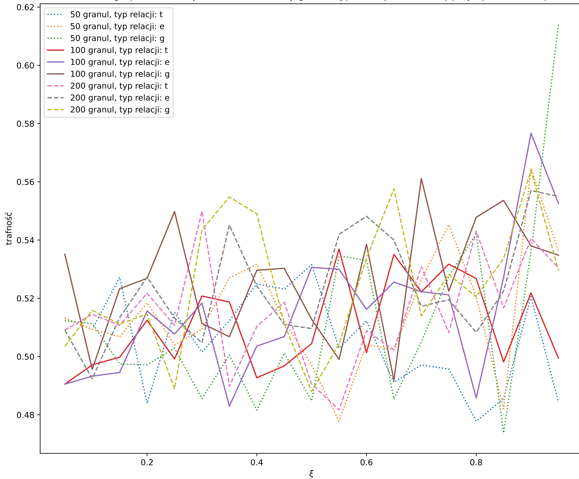
Zależność trafności grupowania danych corners od liczby granul, typu relacji i wartości \xi przy łączności complete linkage
