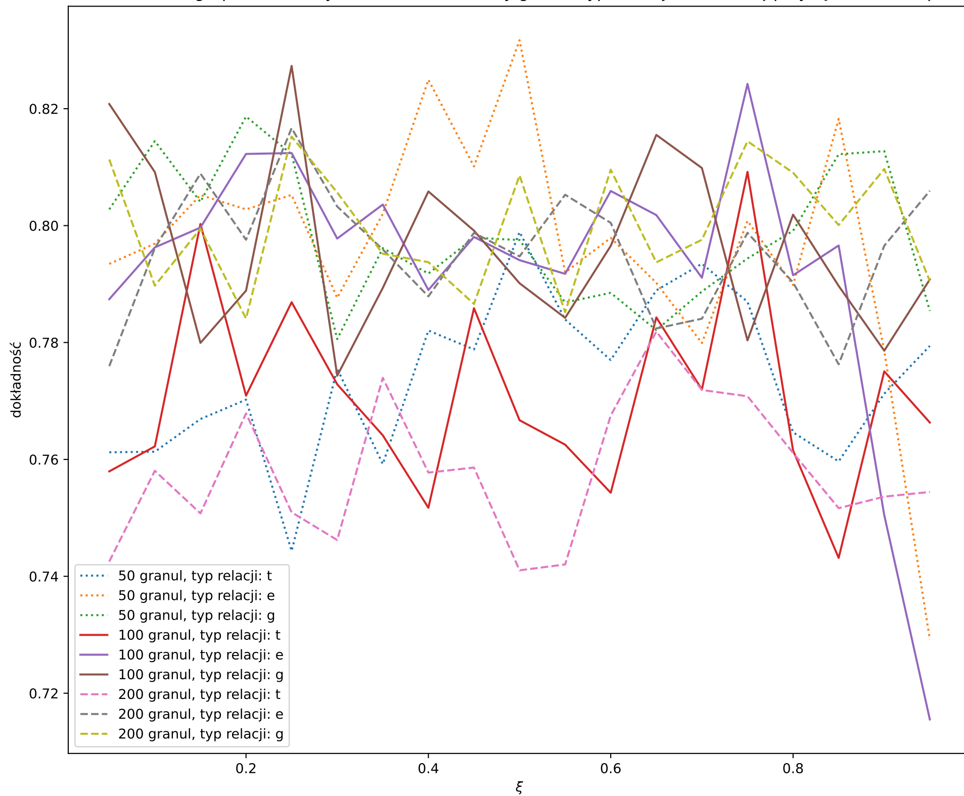
Zależność dokładności grupowania danych crescents od liczby granul, typu relacji i wartości \xi przy łączności complete linkage
