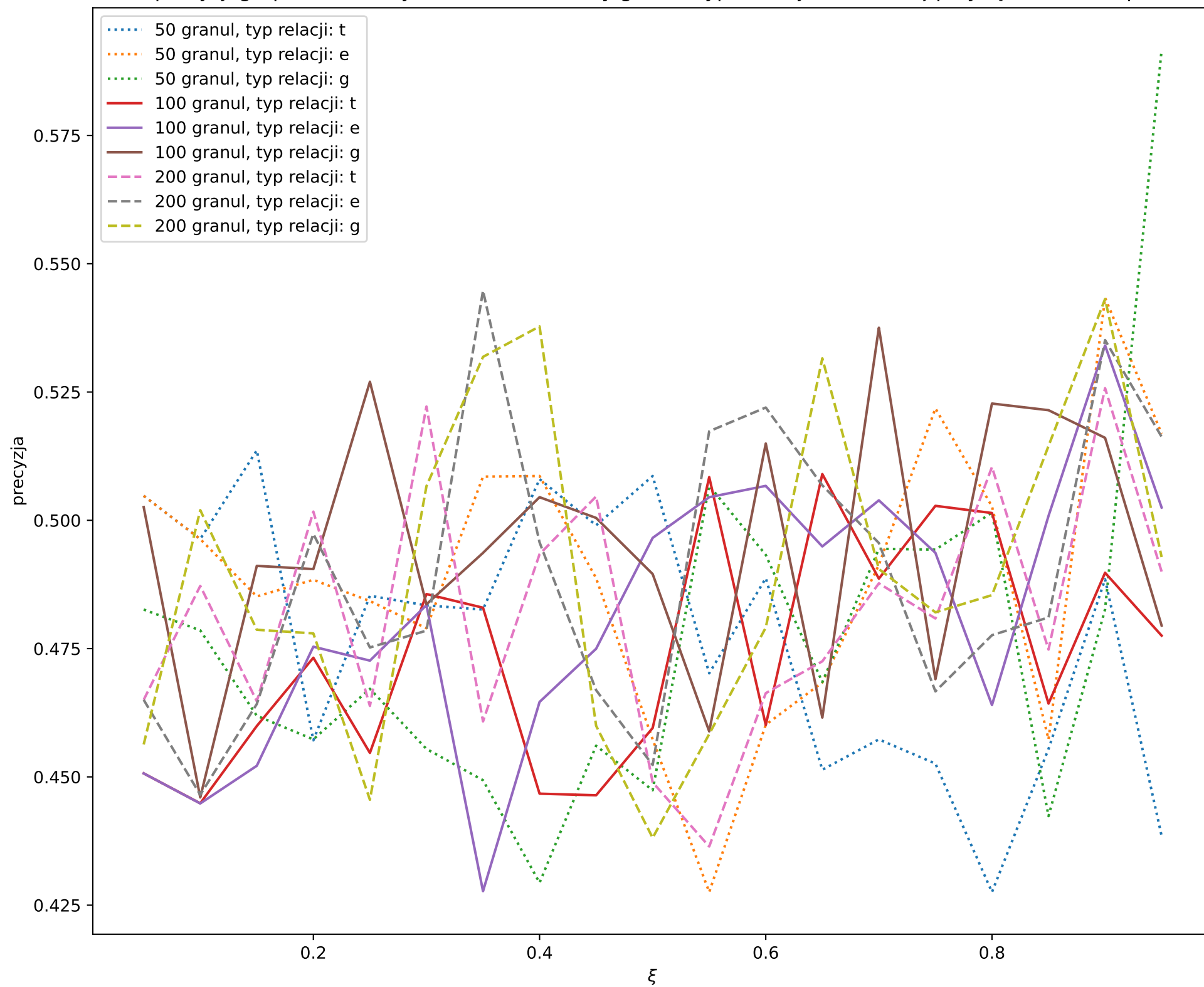
Zależność precyzji grupowania danych corners od liczby granul, typu relacji i wartości \xi przy łączności complete linkage
