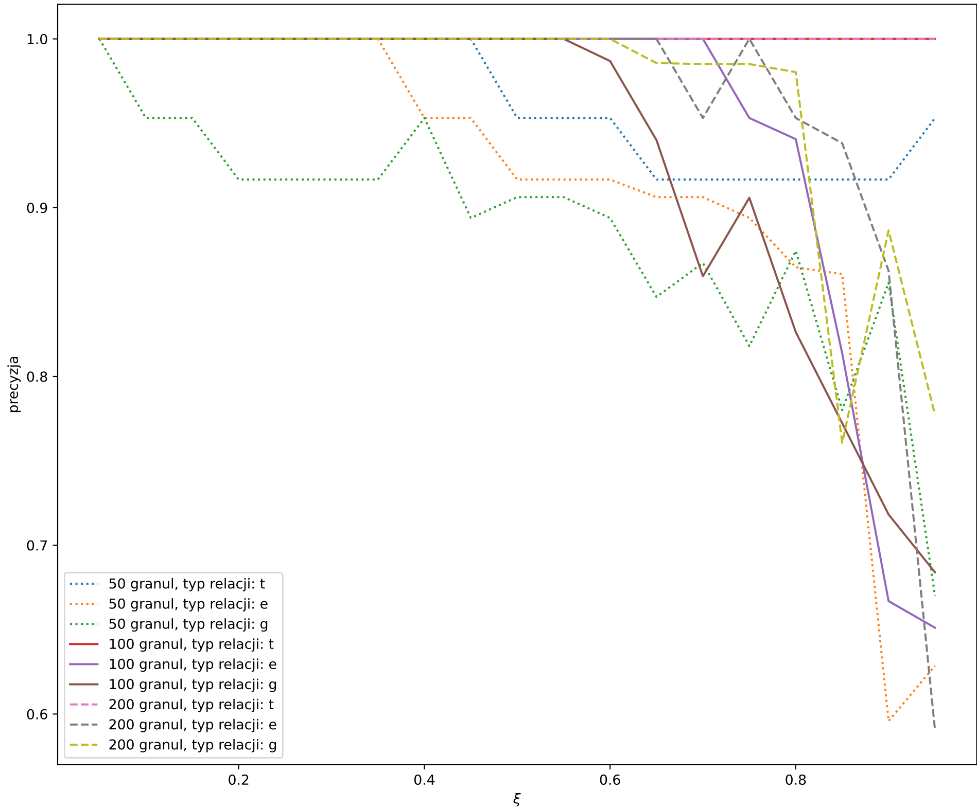
Zależność precyzji grupowania danych corners od liczby granul, typu relacji i wartości \xi przy łączności single linkage
