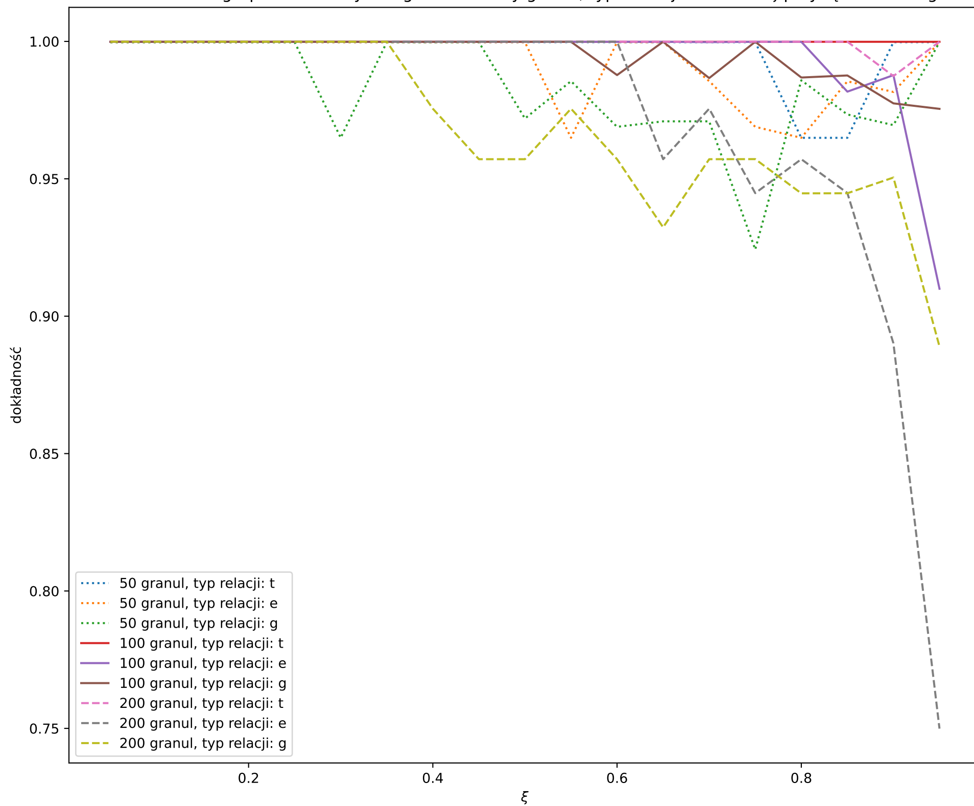
Zależność dokładności grupowania danych laguna od liczby granul, typu relacji i wartości \xi przy łączności single linkage
