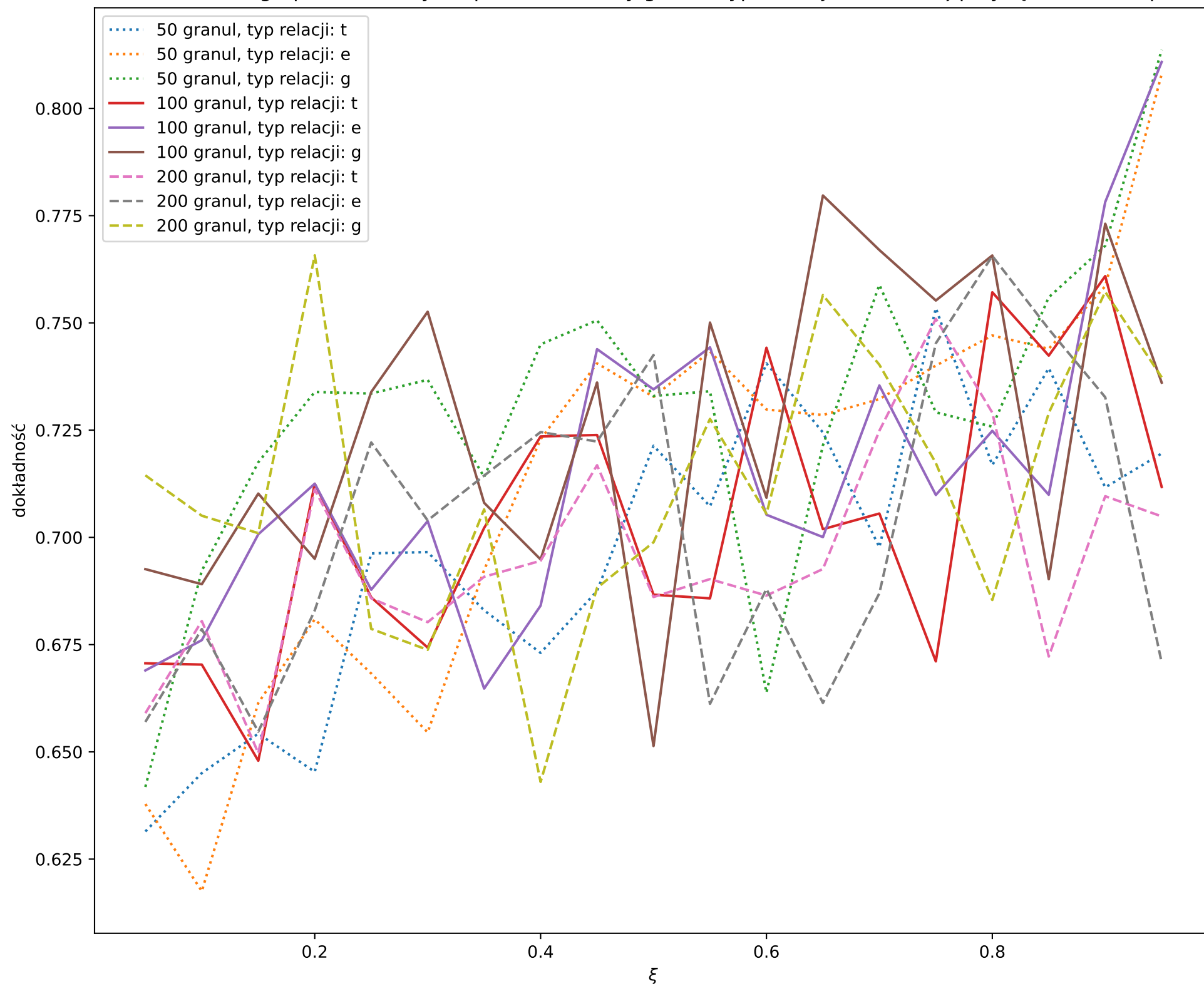
Zależność dokładności grupowania danych spheres od liczby granul, typu relacji i wartości \xi przy łączności complete linkage
