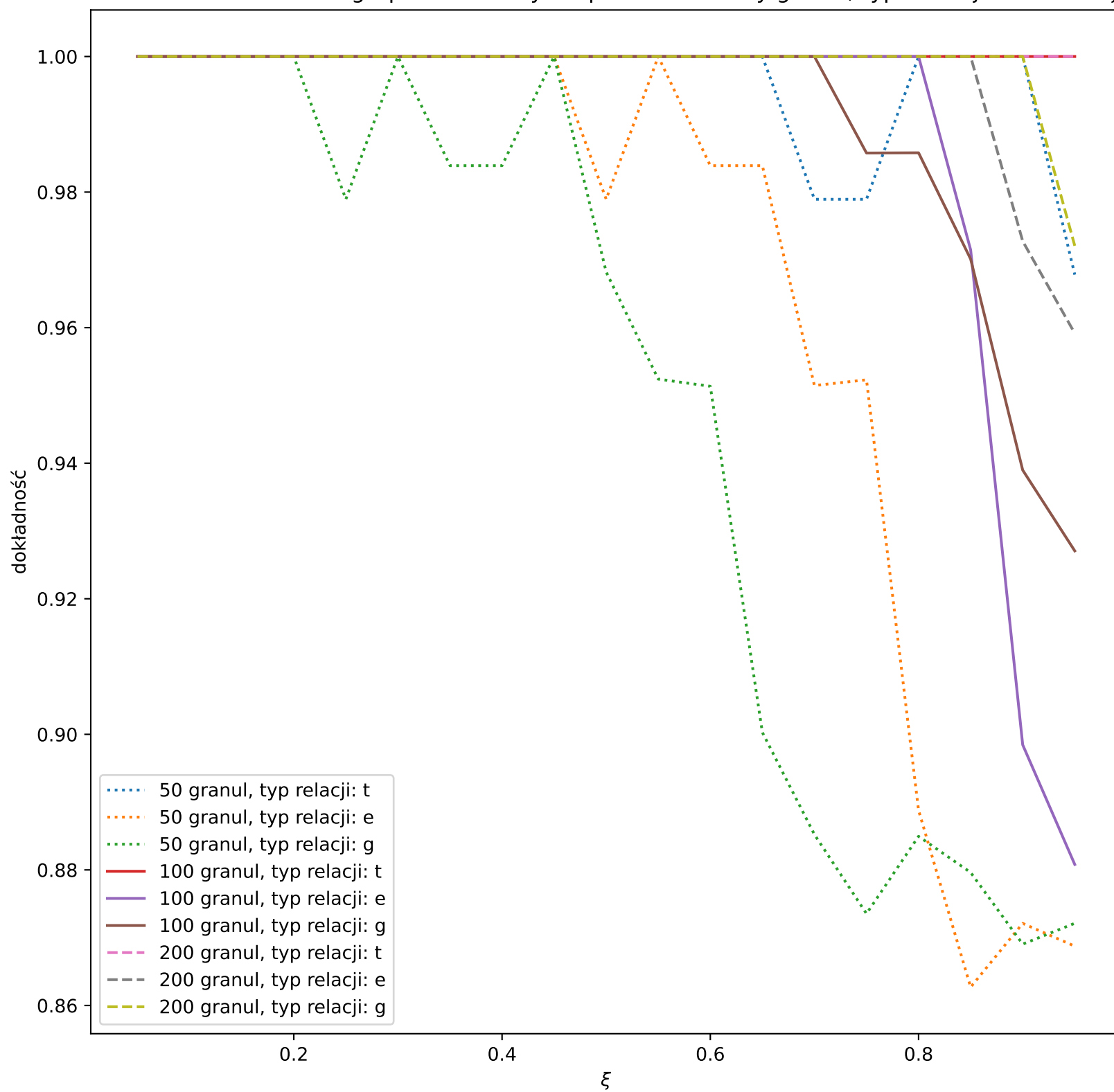
Zależność dokładności grupowania danych spheres od liczby granul, typu relacji i wartości \xi
