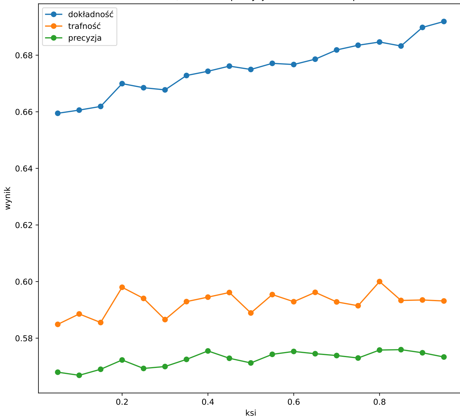
Średnia dokładność, trafność i precyzja w zależności od parametru ksi
