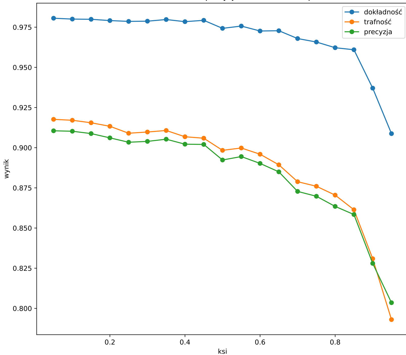
Średnia dokładność, trafność i precyzja w zależności od parametru ksi
