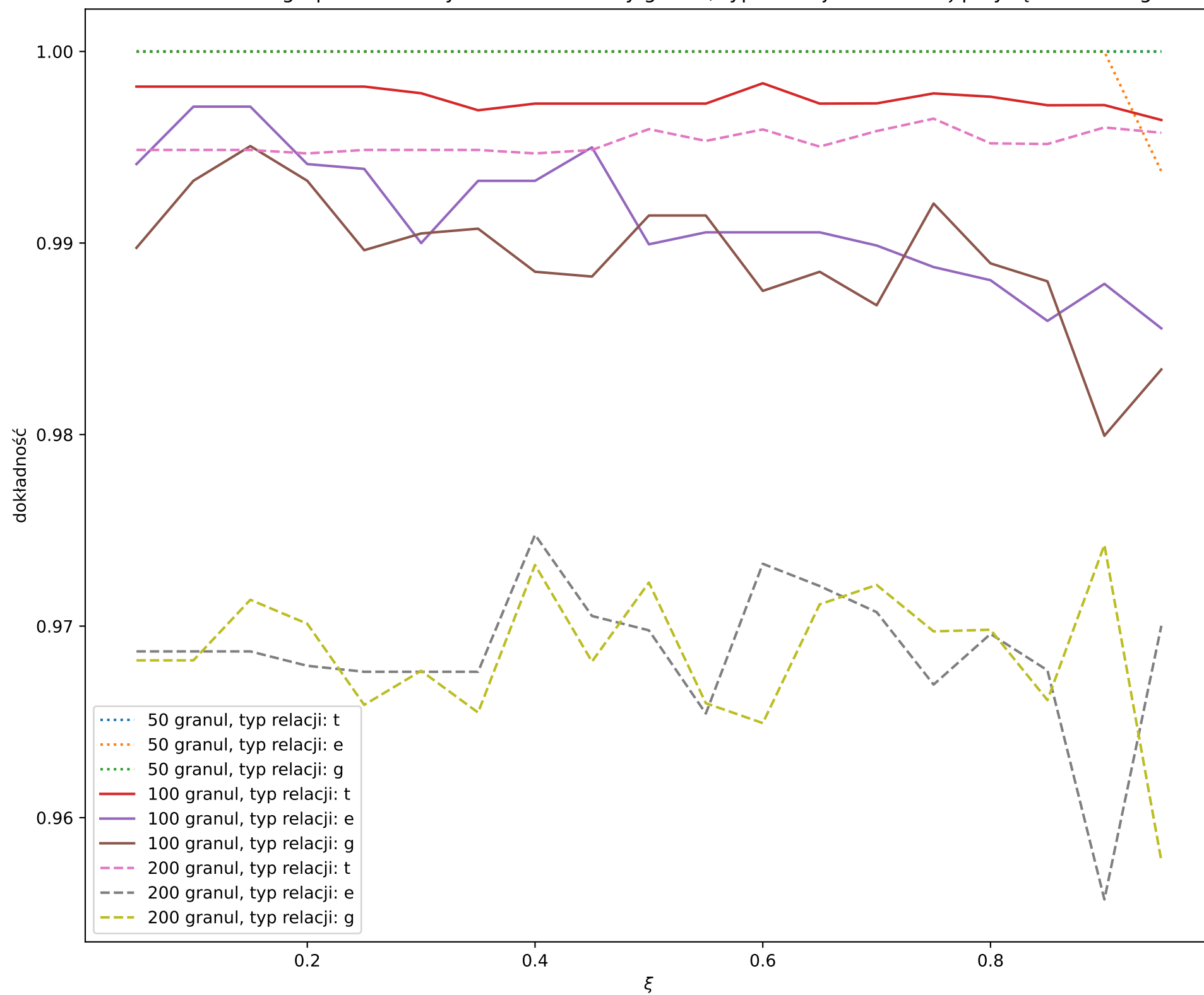
Zależność dokładności grupowania danych blobs od liczby granul, typu relacji i wartości \xi przy łączności single linkage
