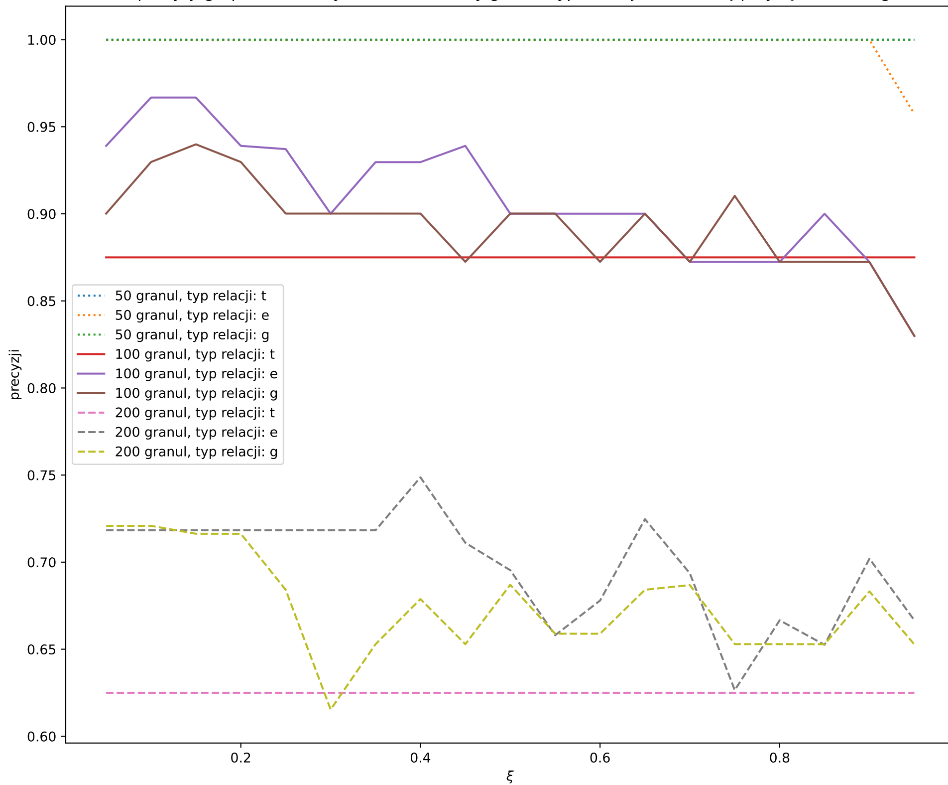
Zależność precyzji grupowania danych blobs od liczby granul, typu relacji i wartości \xi przy łączności single linkage
