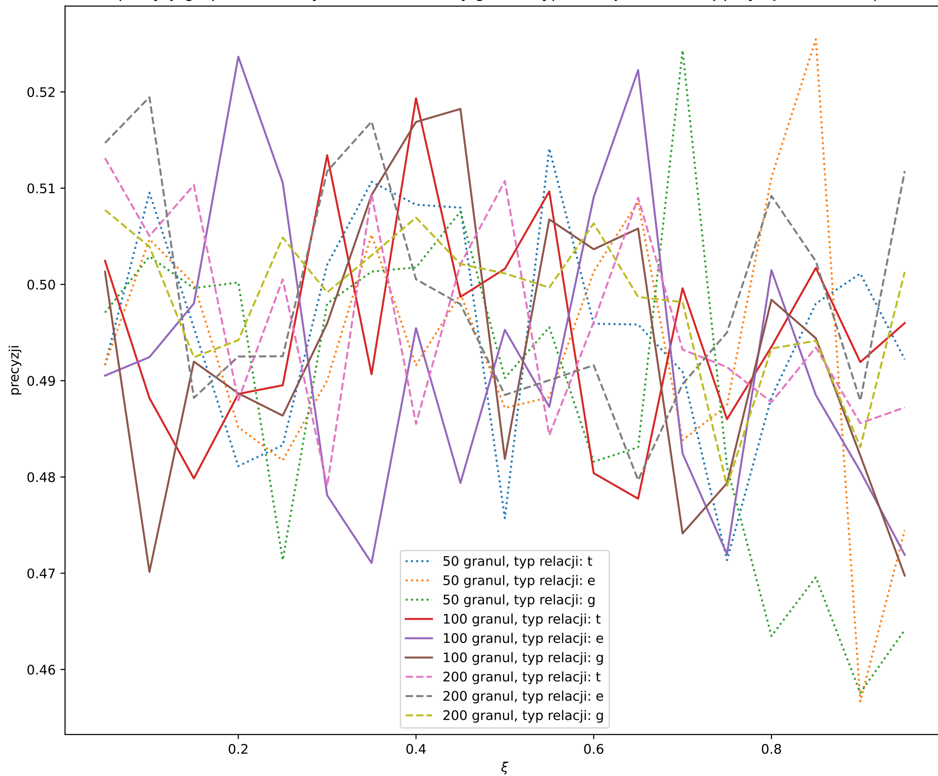
Zależność precyzji grupowania danych circles od liczby granul, typu relacji i wartości \xi przy łączności complete linkage
