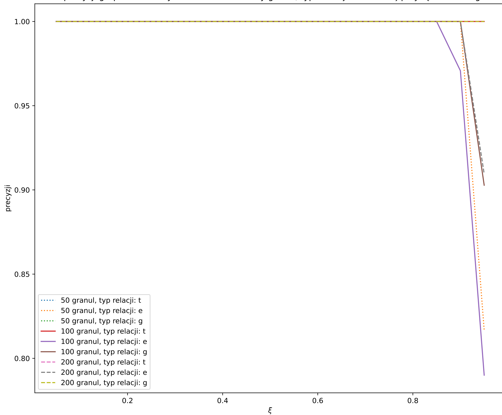
Zależność precyzji grupowania danych crescents od liczby granul, typu relacji i wartości \xi przy łączności single linkage
