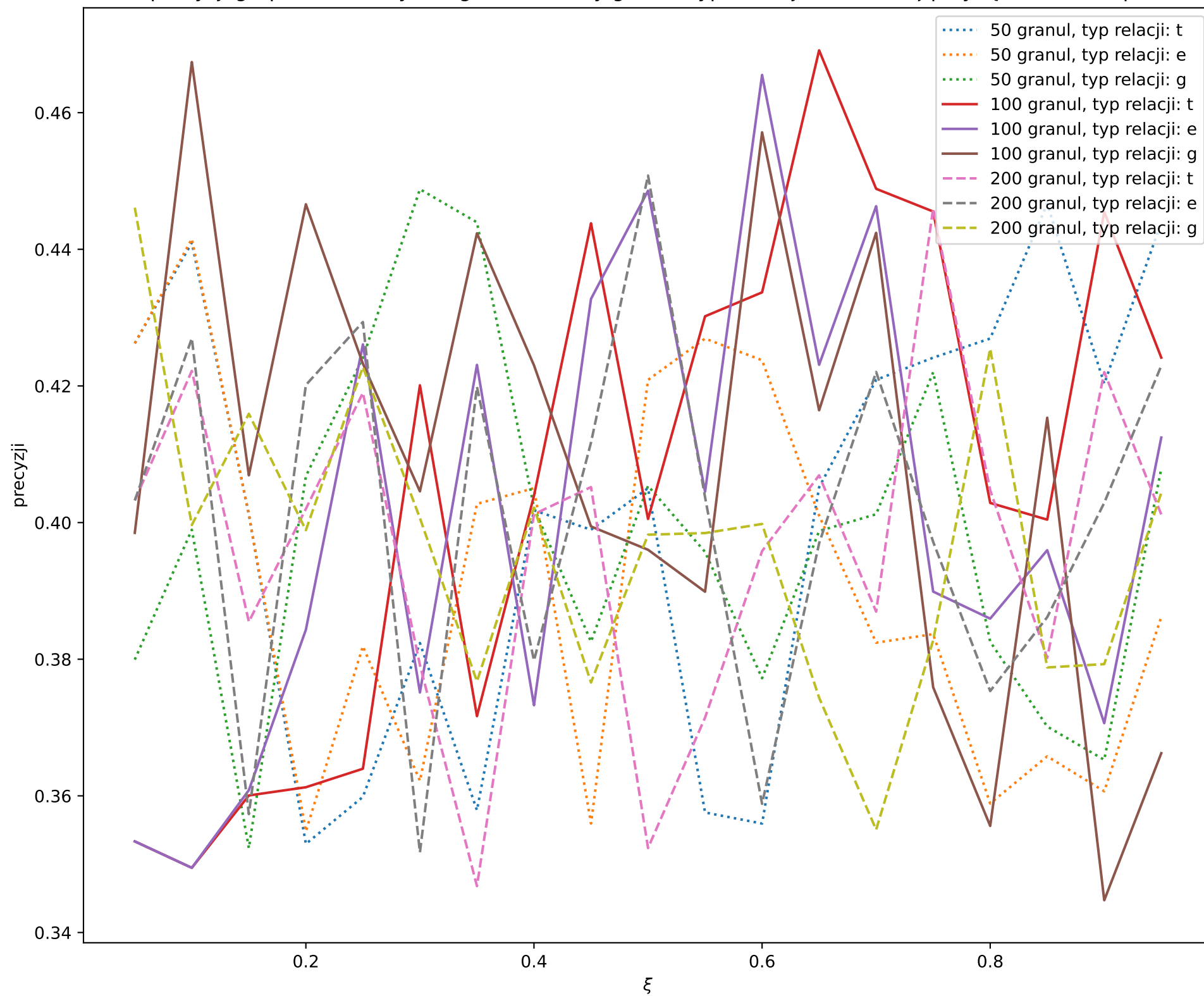
Zależność precyzji grupowania danych laguna od liczby granul, typu relacji i wartości \xi przy łączności complete linkage
