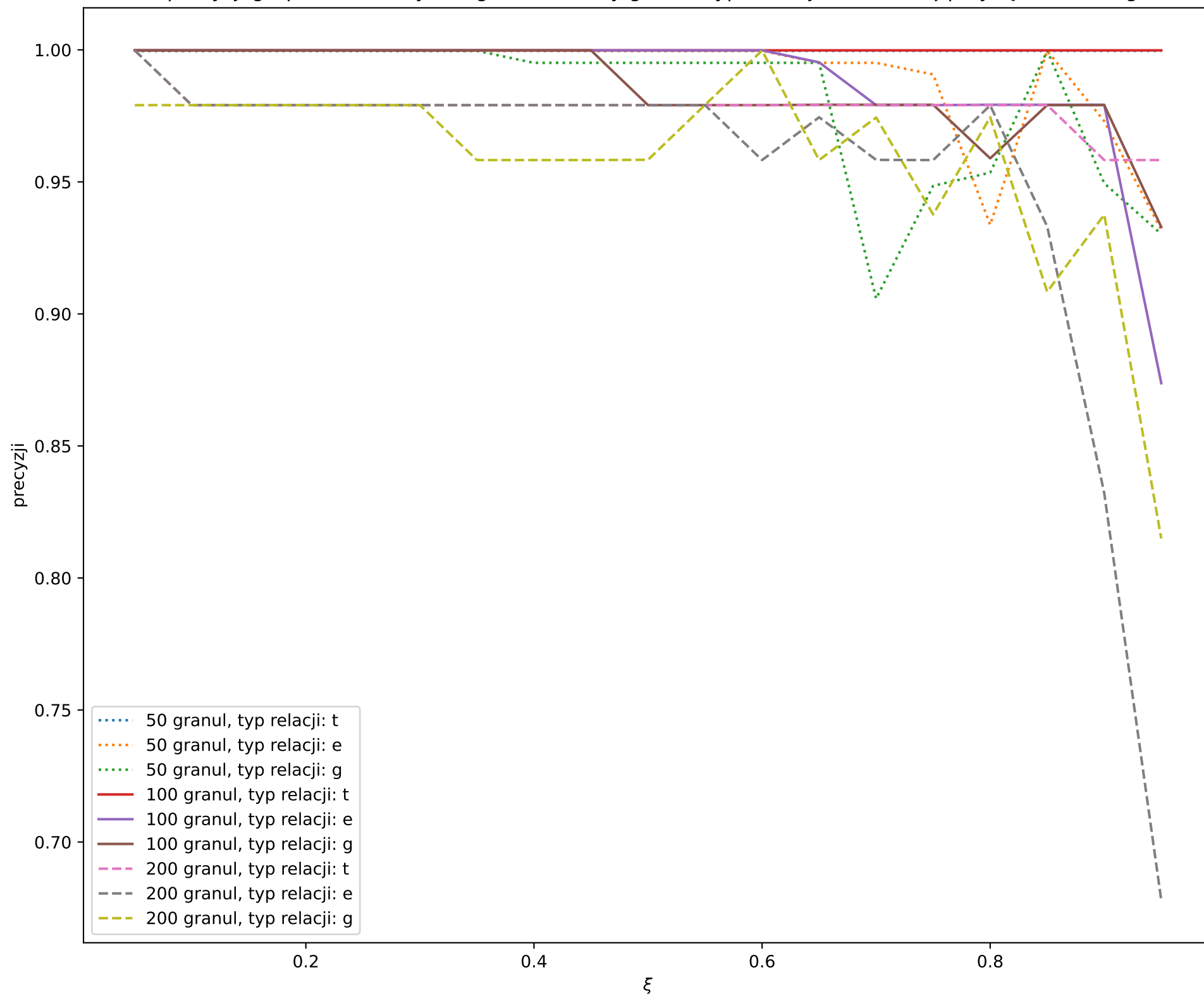
Zależność precyzji grupowania danych laguna od liczby granul, typu relacji i wartości \xi przy łączności single linkage
