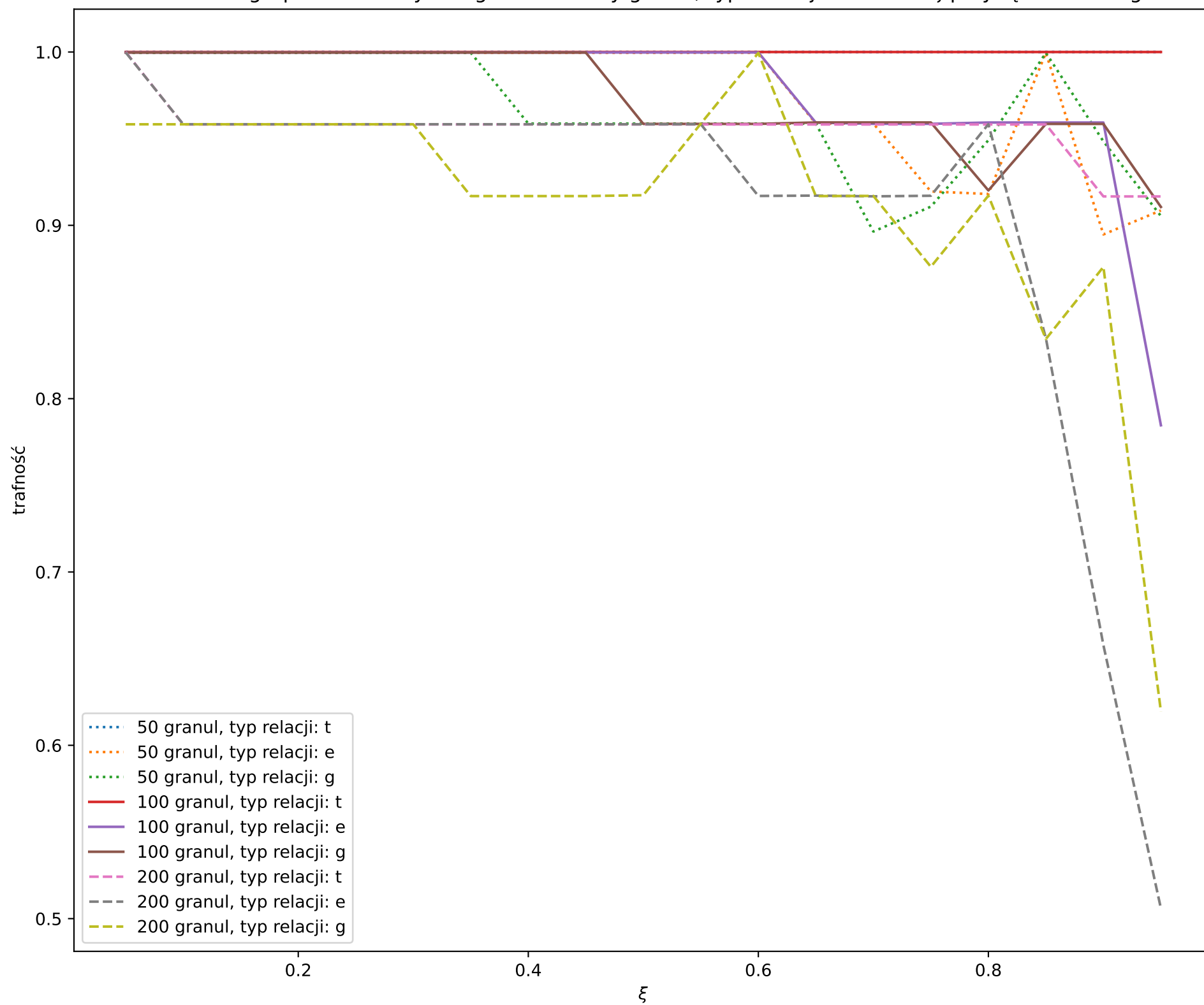
Zależność trafności grupowania danych laguna od liczby granul, typu relacji i wartości \xi przy łączności single linkage
