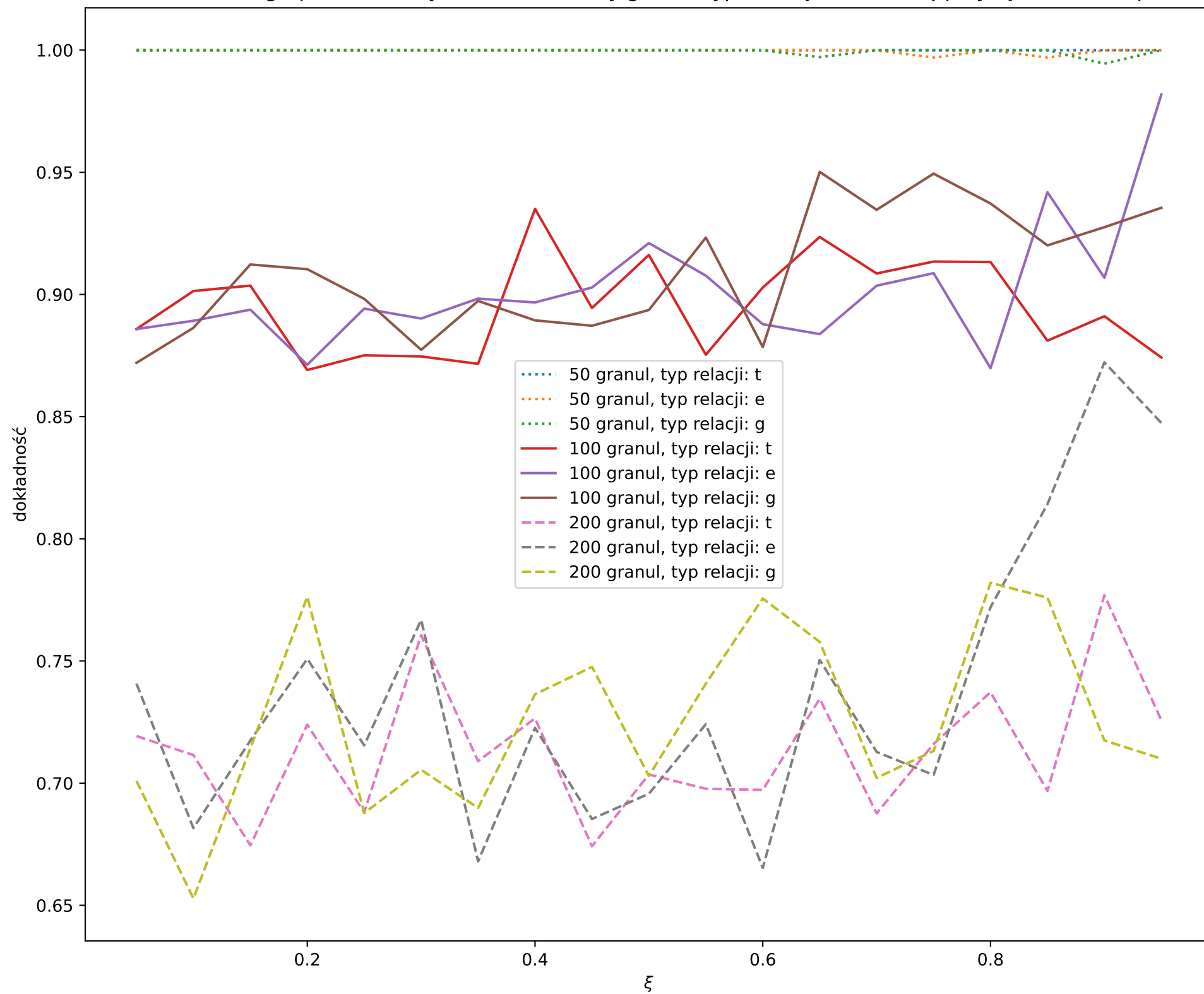
Zależność dokładności grupowania danych blobs od liczby granul, typu relacji i wartości \xi przy łączności complete linkage
