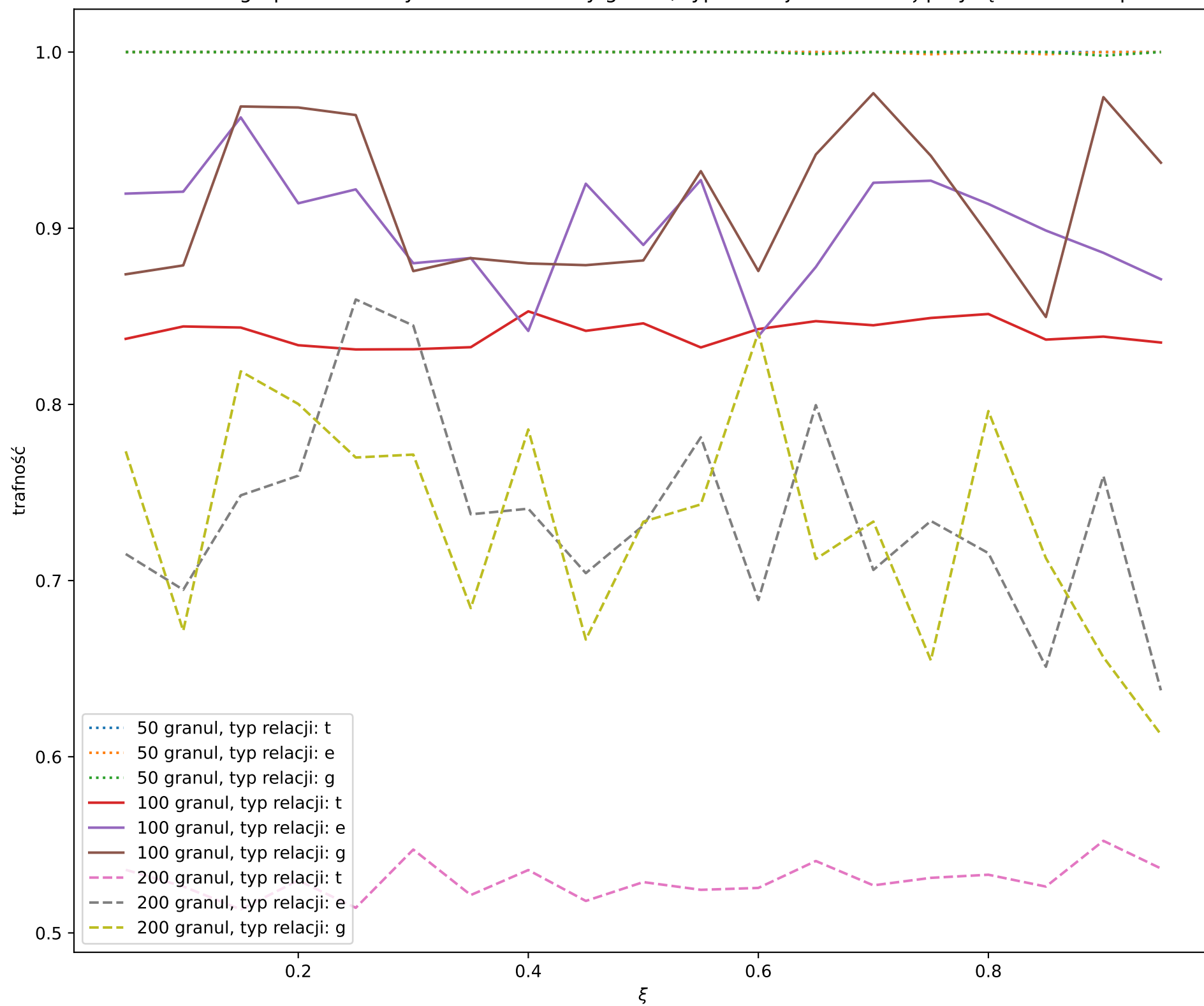
Zależność trafności grupowania danych blobs od liczby granul, typu relacji i wartości \xi przy łączności complete linkage
