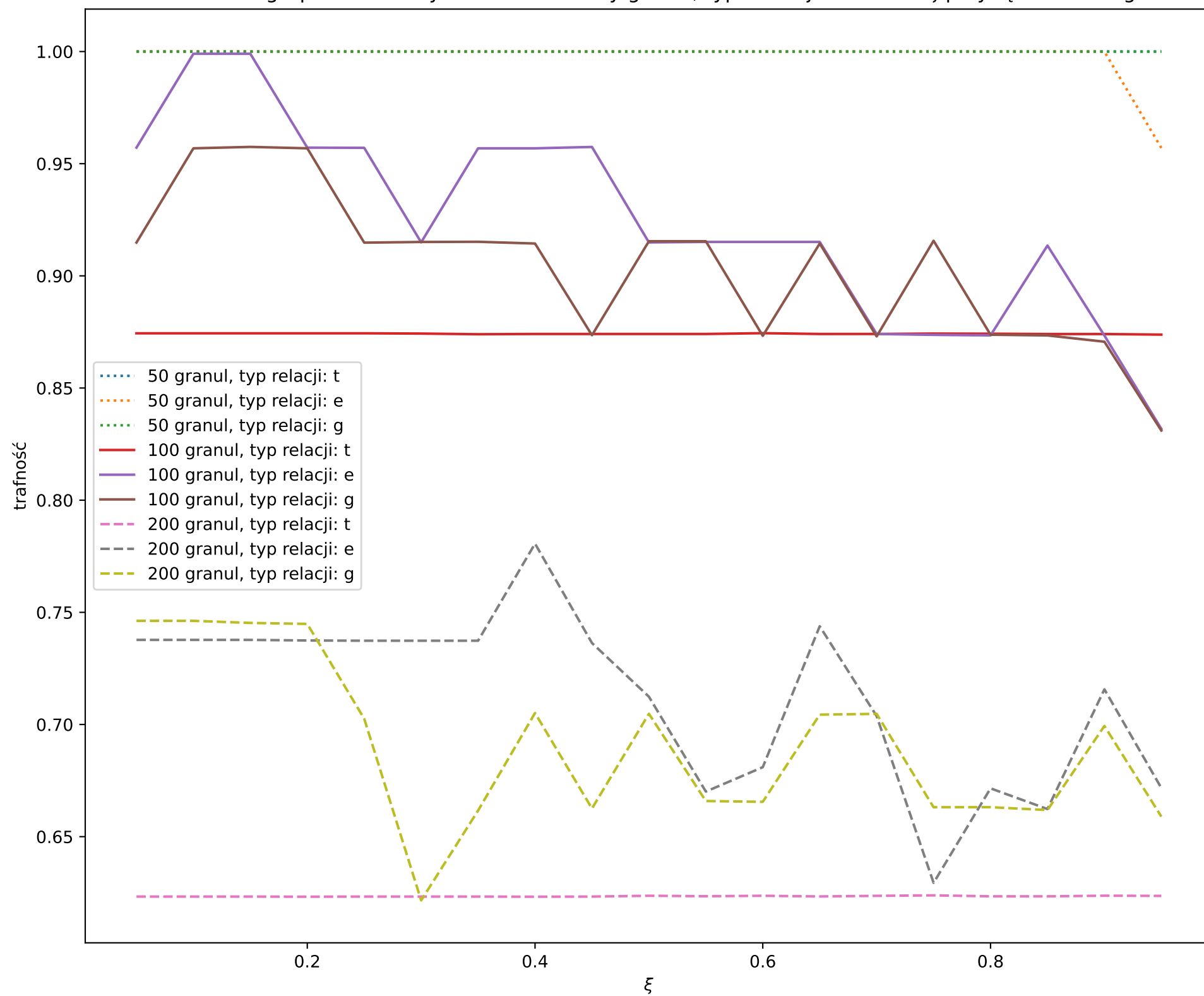
Zależność trafności grupowania danych blobs od liczby granul, typu relacji i wartości \xi przy łączności single linkage
