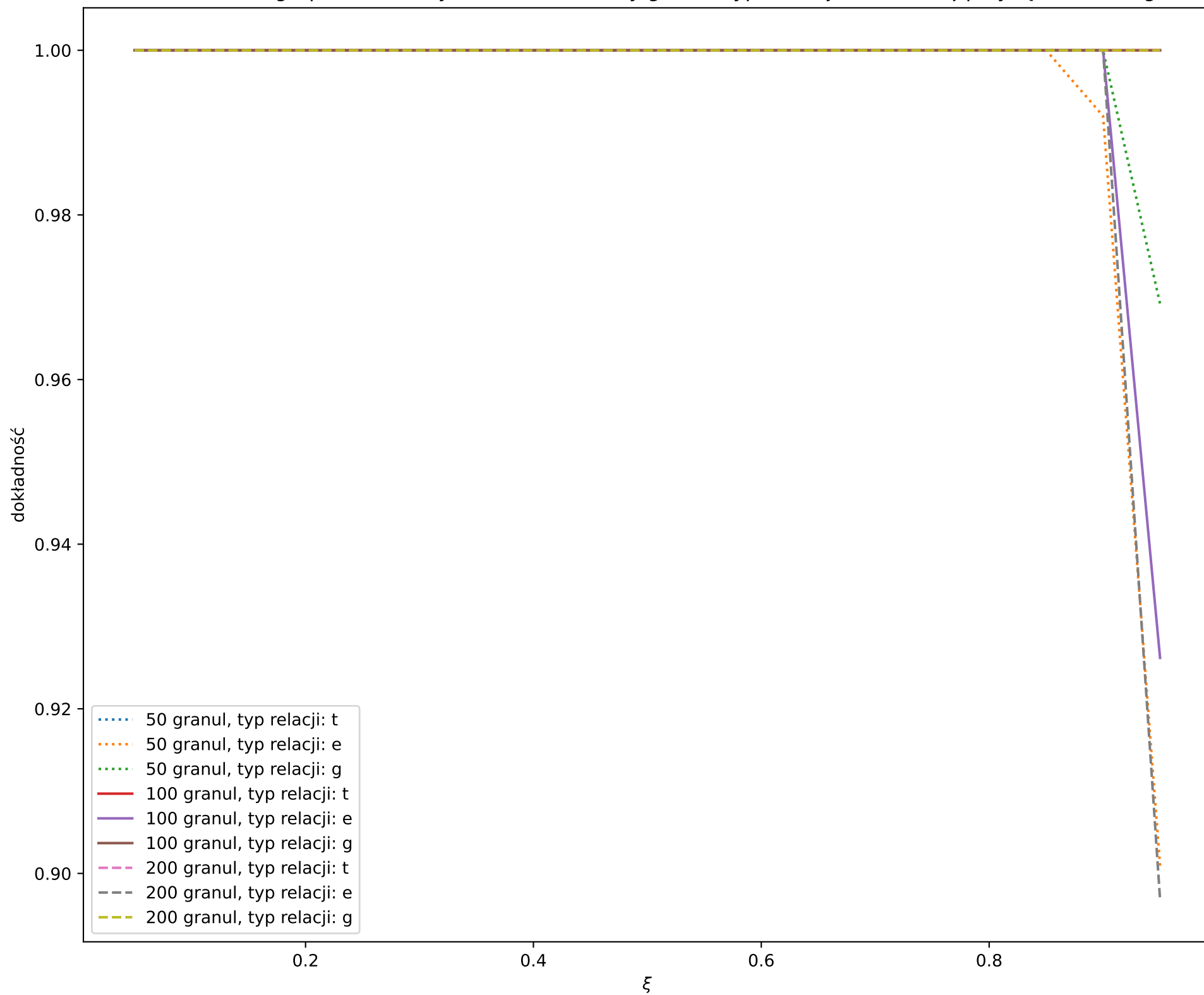
Zależność dokładności grupowania danych circles od liczby granul, typu relacji i wartości \xi przy łączności single linkage
