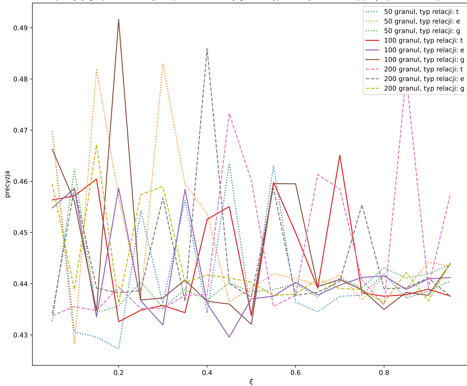
Zależność precyzji grupowania danych spheres od liczby granul, typu relacji i wartości \xi przy łączności complete linkage
