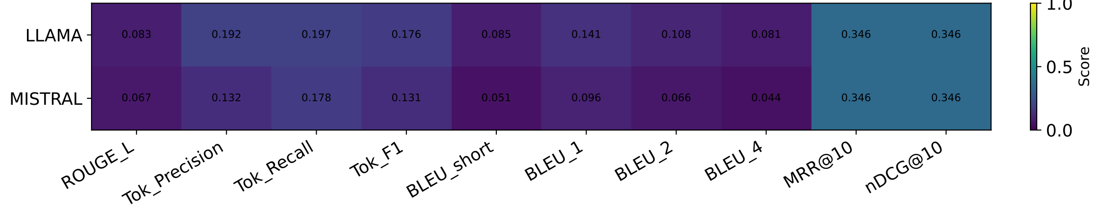
Extra Metrics Heatmap (0-1)
