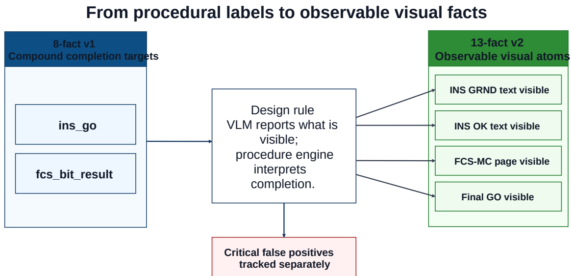
Abbildung 4.2: 从 8 事实 v1 到 13 事实 v2 的本体论演化。诸如 ins_go 和宽泛的 FCS-MC 完成事实等复合目标被分解为局部可验证的视觉原子；程序引擎随后将这些观察与遥测、阶段和时序证据相结合。
