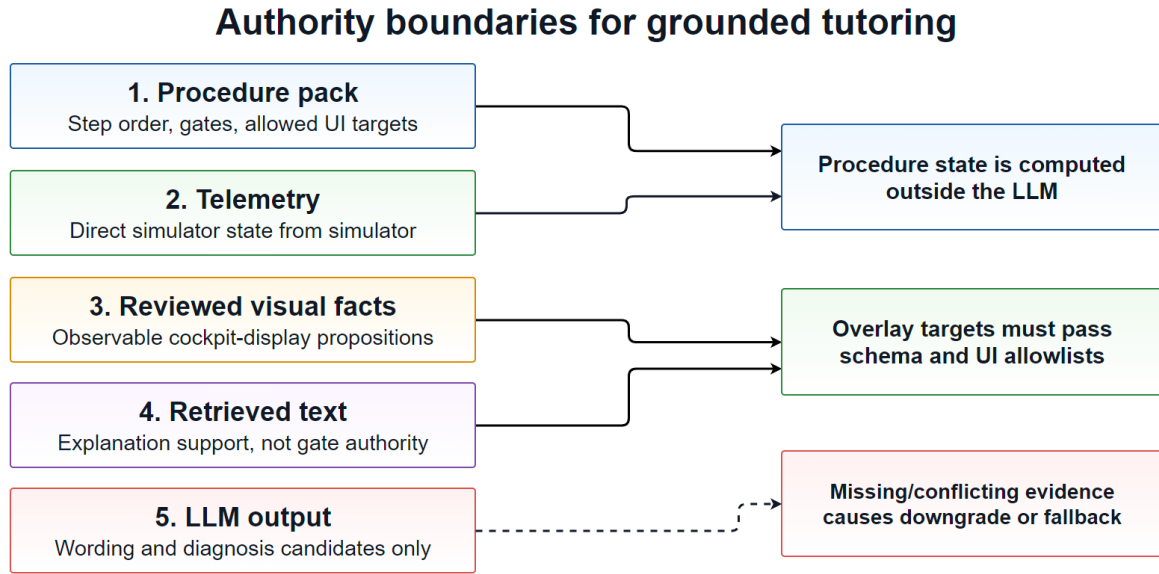
Abbildung 3.2: 基于证据的教学的权威边界。程序规则和遥测约束状态；审查过的视觉事实提供有边界的显示证据；检索和 LLM 输出支持解释但不覆盖门禁条件或 UI 白名单。
