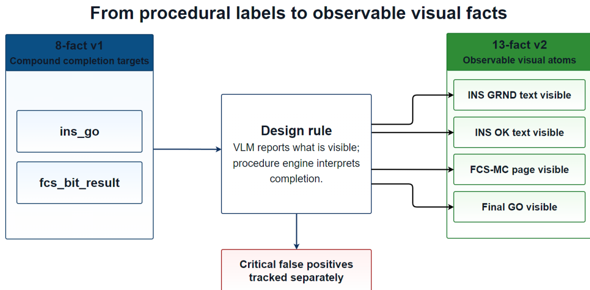
Abbildung 4.2: 从 8 事实 v1 到 13 事实 v2 的本体论演化。诸如 ins_go 和宽泛的 FCS-MC 完成事实等复合目标被分解为局部可验证的视觉原子；程序引擎随后将这些观察与推测、阶段和时序证据相结合。
