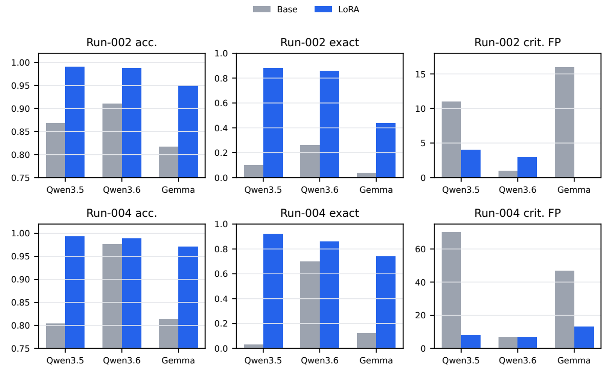
Abbildung 6.3: Qwen3.5、Qwen3.6 和 Gemma 在 Run-003 + Run-005×2 方案下的匹配骨干模型比较。面板分别报告 Run-002 和 Run-004 上的事实准确率、完全匹配率和关键假阳性计数。
