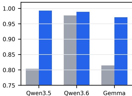
Run-004 acc.
