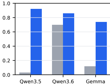
Run-004 exact
