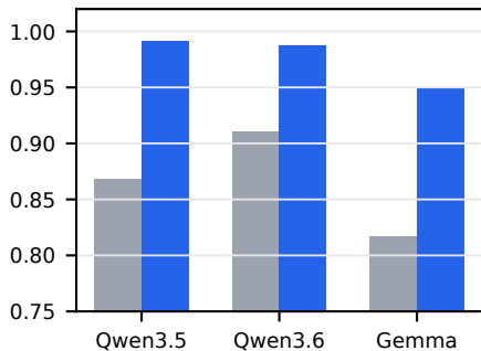
Run-004 acc.
