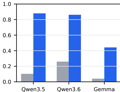
Run-002 exact
