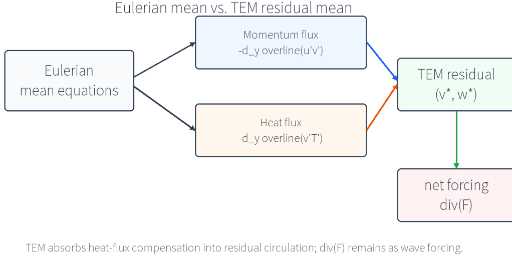
图 1: 传统 Eulerian 平均与 TEM 的诊断差异。TEM 将热通量辐合与绝热冷却的近似抵消显式化, 留下 \nabla \cdot \mathbf{F} 作为波对平均流的合成强迫。
