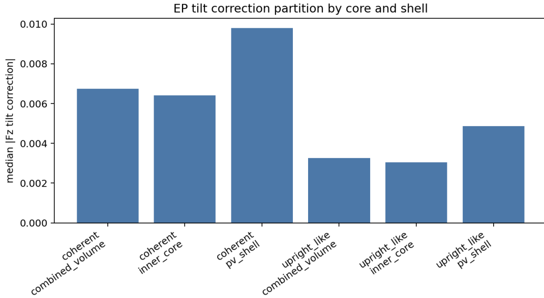
图 9: EP tilt correction 的 core-shell 分区。倾斜修正与 PV-active shell 和交换带联系更强，支持 Dual-Zone 而不是单一材料体解释。
