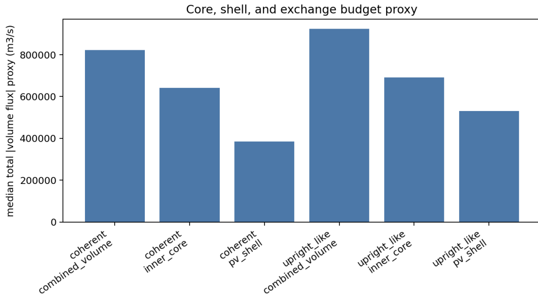
图 10: Core-shell exchange budget。该图体现 exchange layer 的物理角色：它不是误差项，而是材料核与 PV-active shell 之间真实交换的诊断账户。
