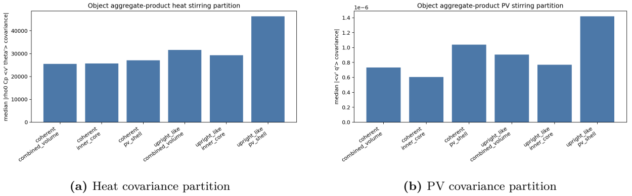
图 8: 热/PV stirring 的 core-shell 分区。PV 通量更明显偏 shell, 说明 PV-active shell 是动力搅拌的重要区域。
