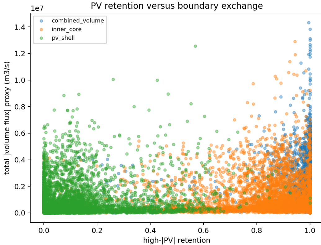
图 6: PV retention 与 boundary exchange 对照。该图支持一个关键判断：PV-active 区域并不总在低泄漏 LAVD/material core 内部。
