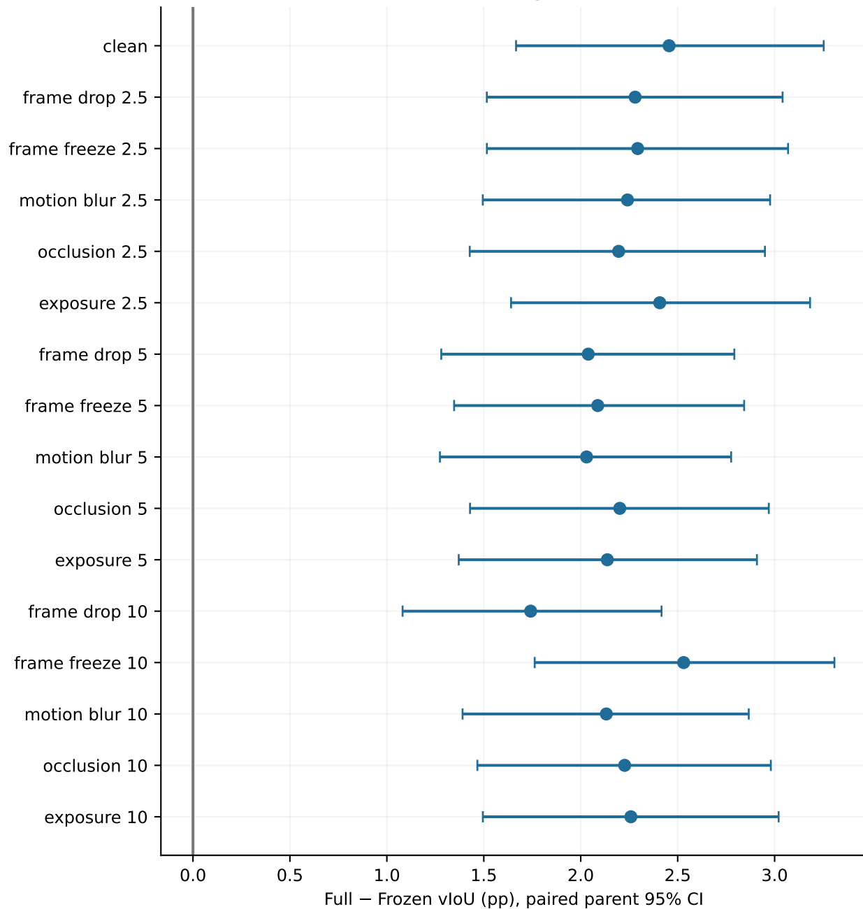
vidstg
