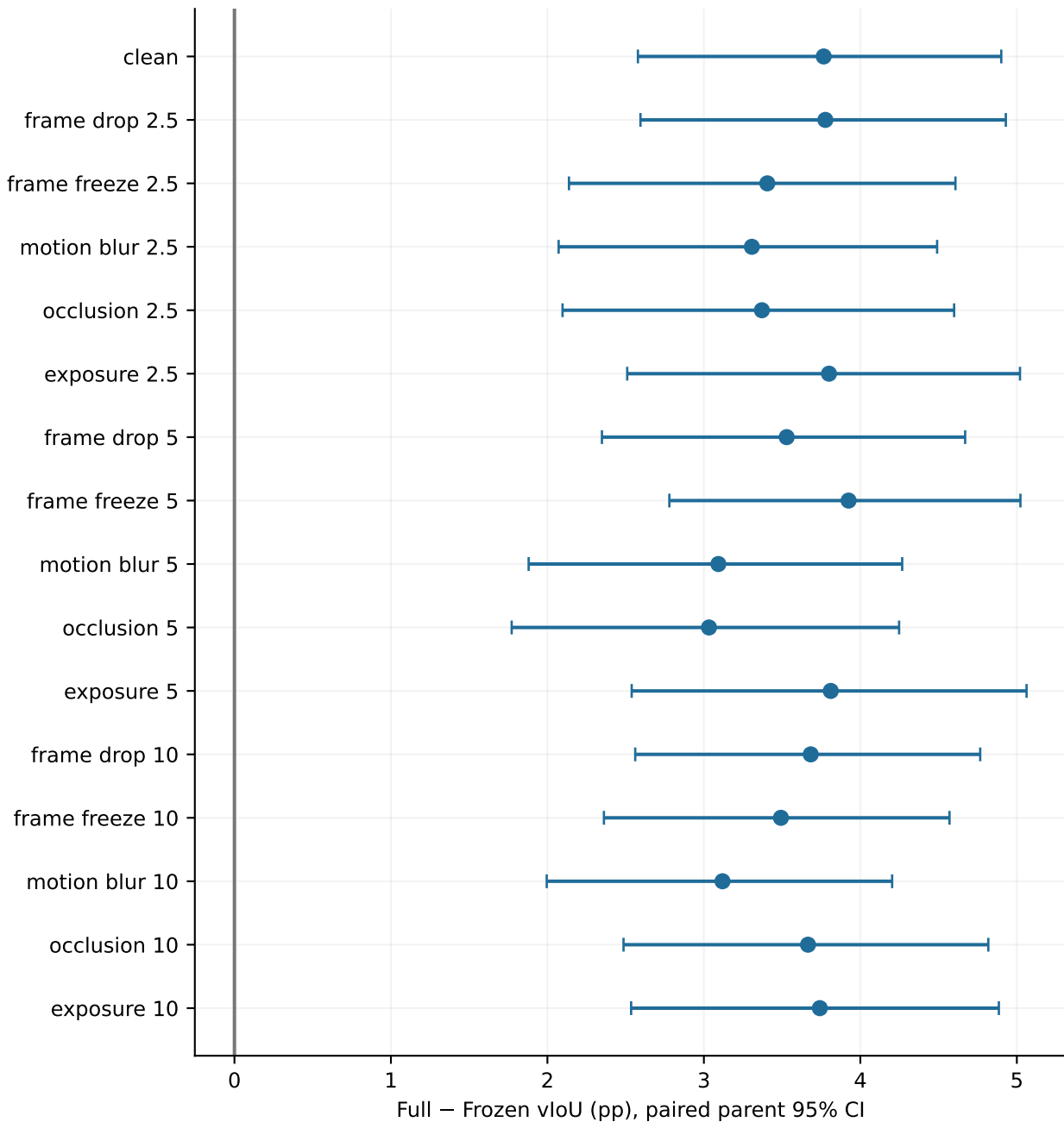
hc2
