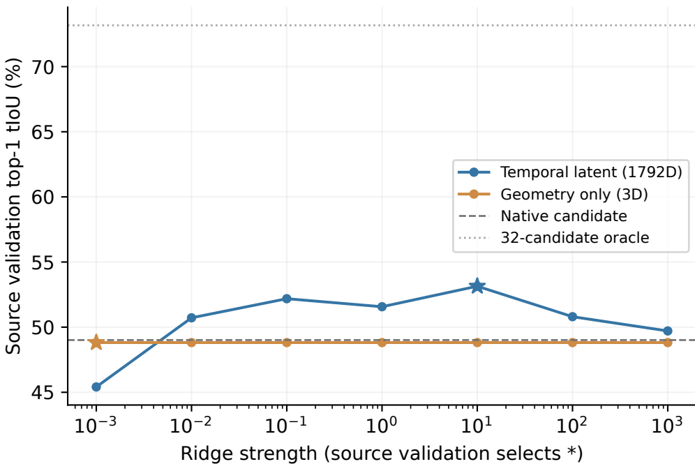
VidSTG
