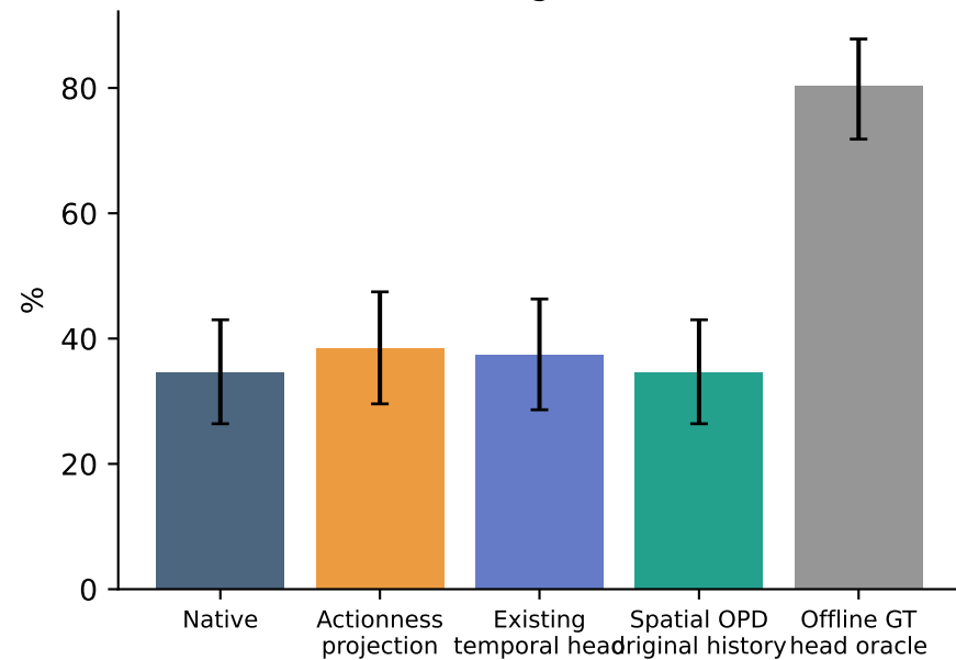
vidstg tIoU
