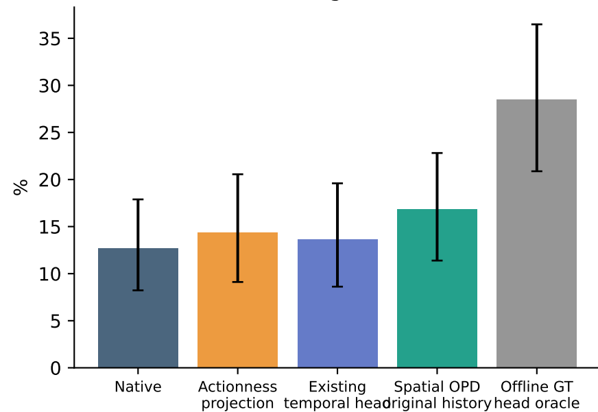
vidstg vIoU
