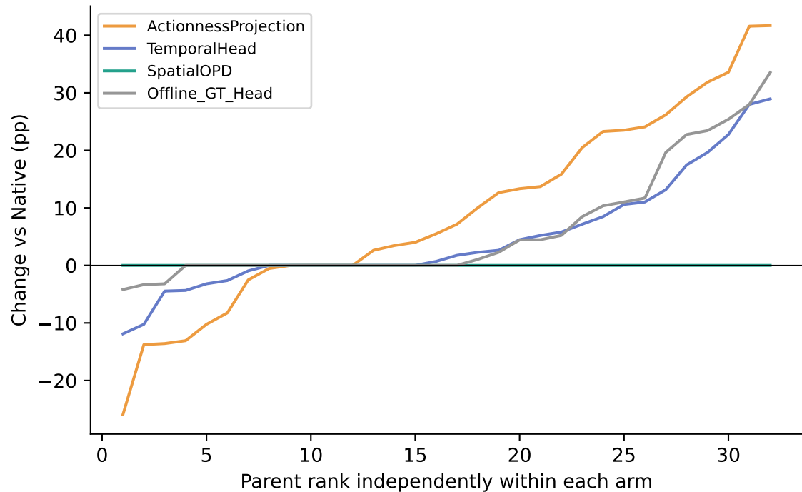
vidstg tIoU complete parent effects
