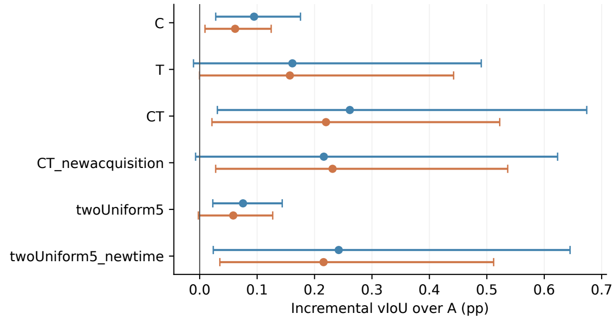
VidSTG
