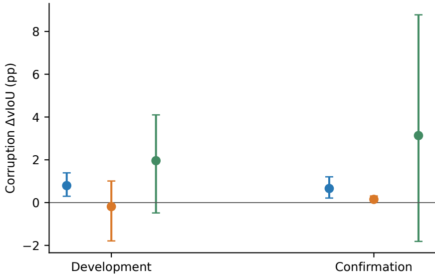
VidSTG
