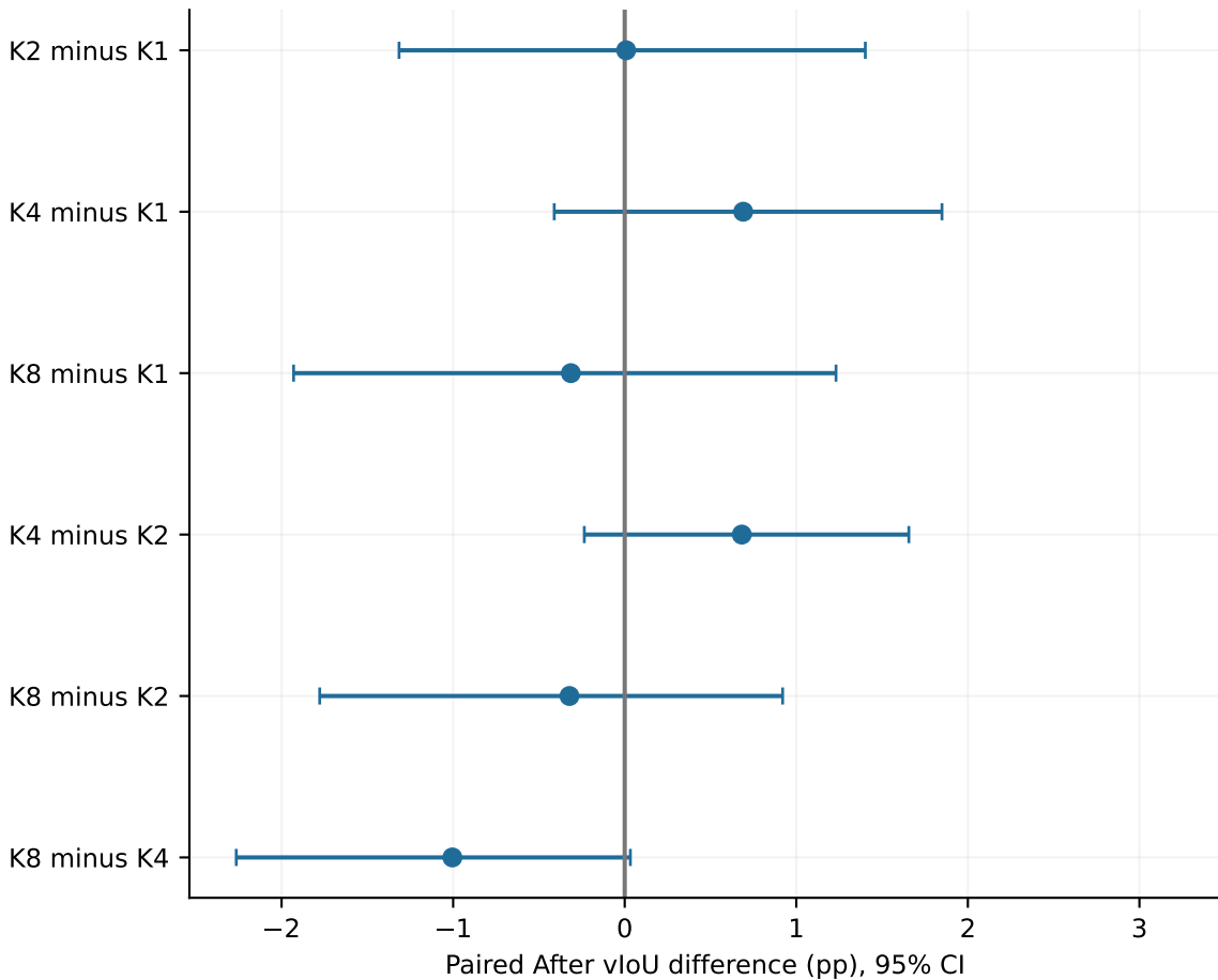
hc2
