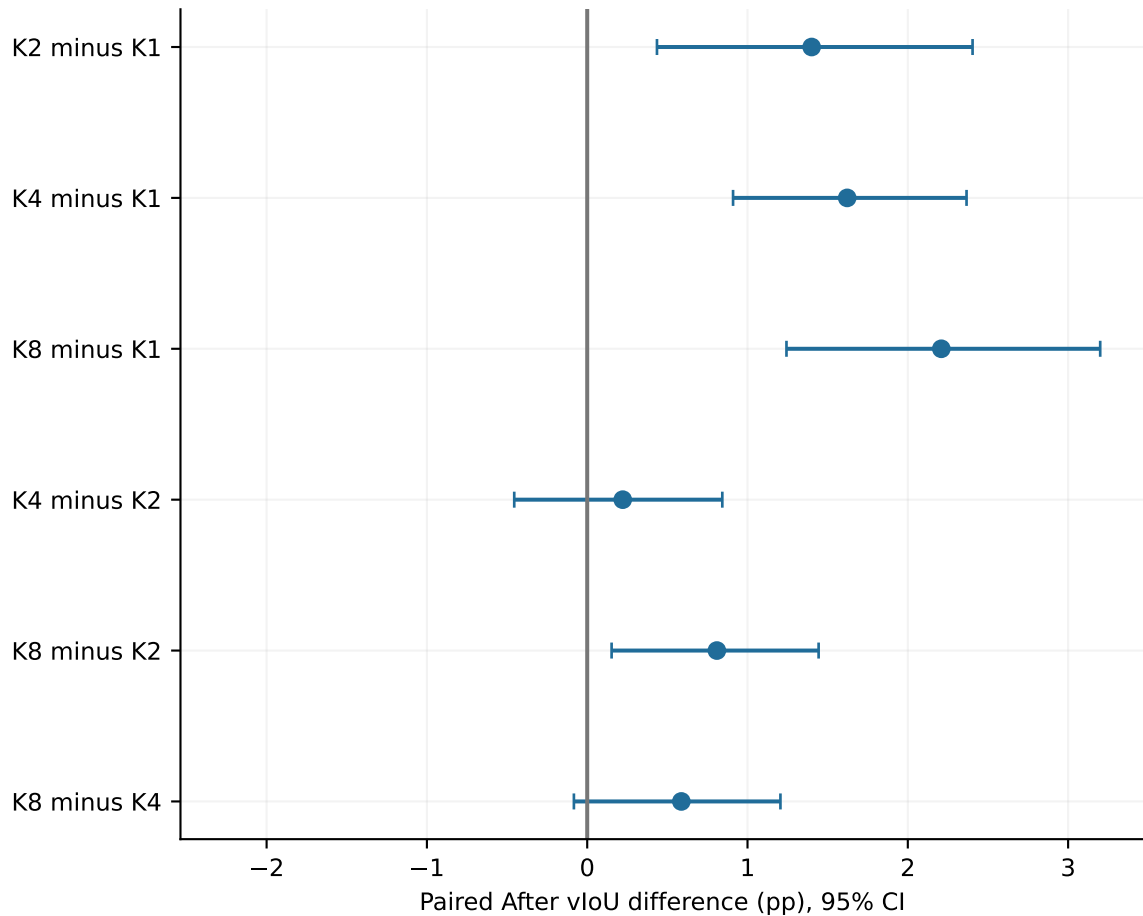
vidstg
