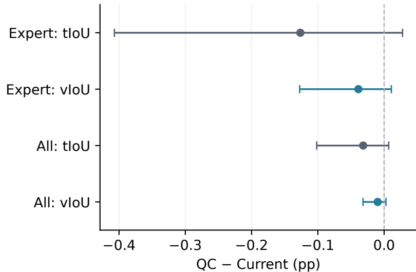
VidSTG
