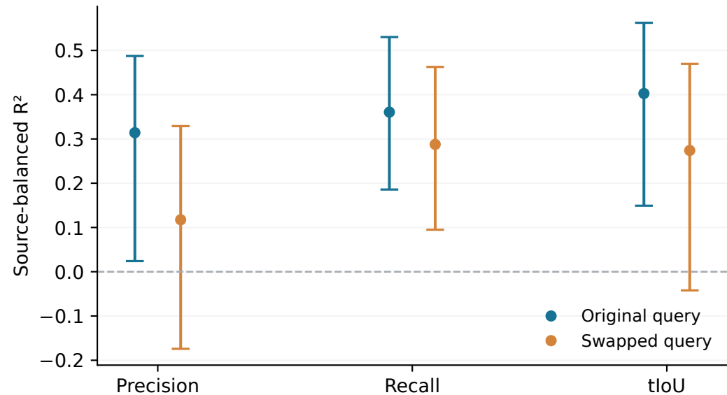
VidSTG
