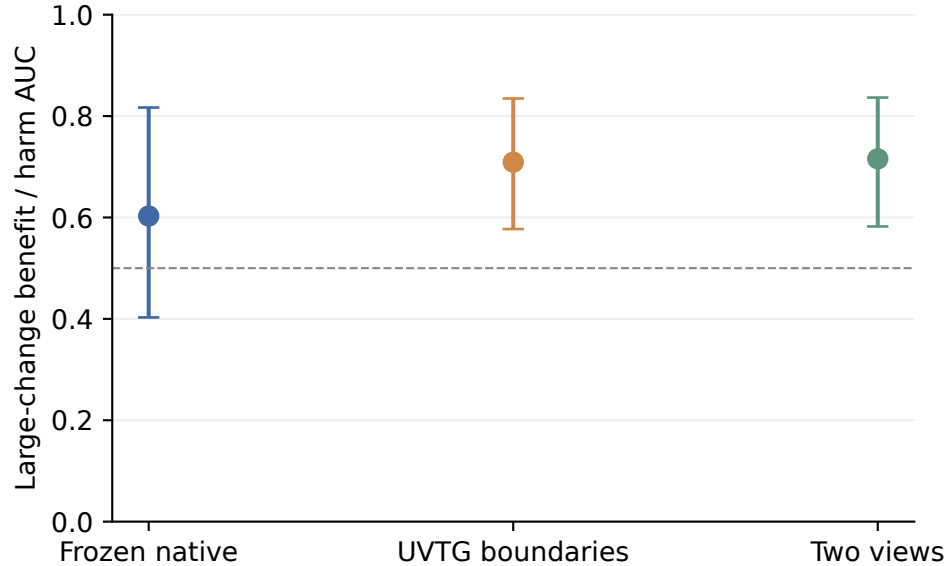
VidSTG
