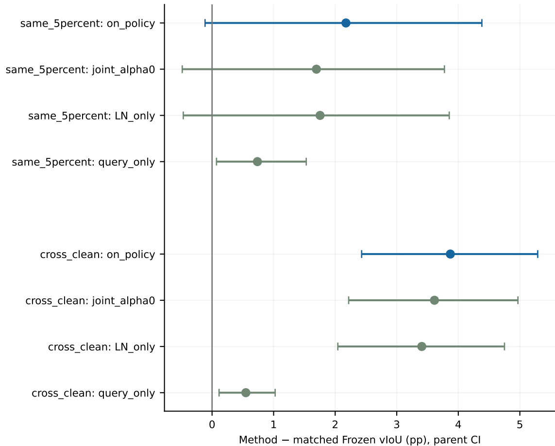
vidstg P3
