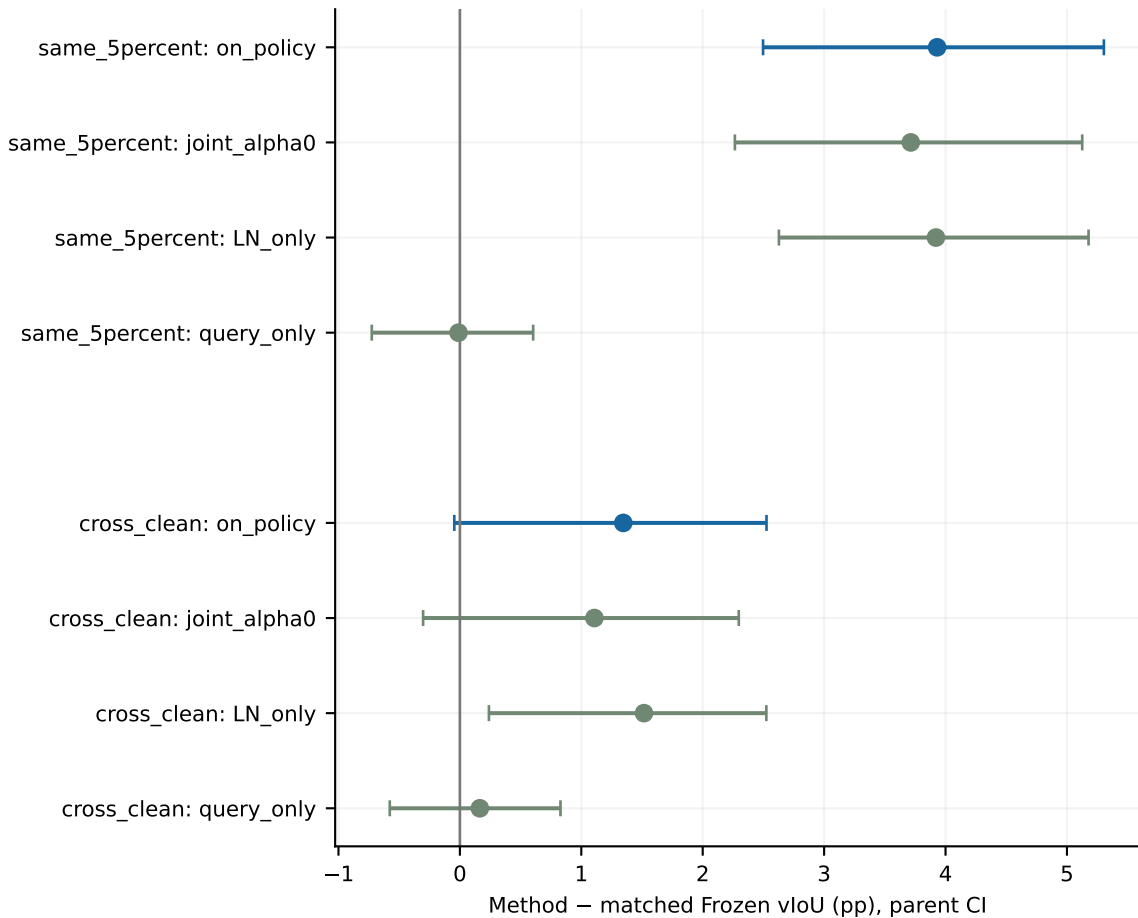
hc2 P3
