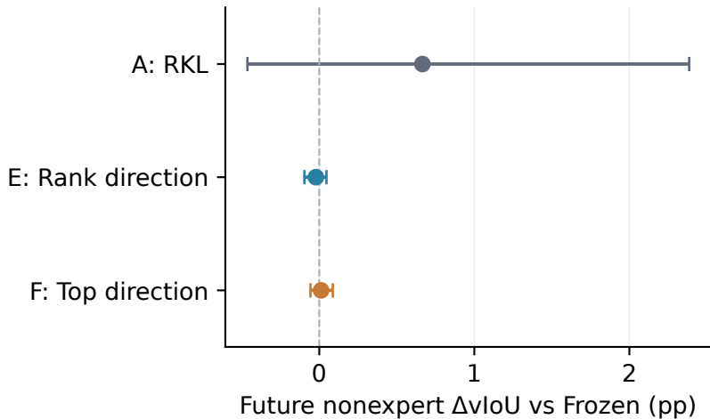
VidSTG
