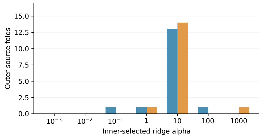
VidSTG · R head
