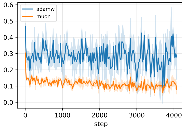
(e) \cos(\text{update}, -\text{gradient})
