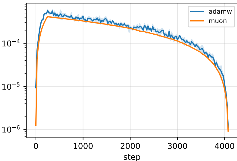
(d) update size per step
