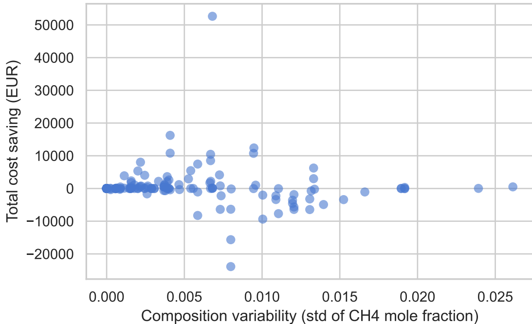
Cost saving vs LNG compositional variability
