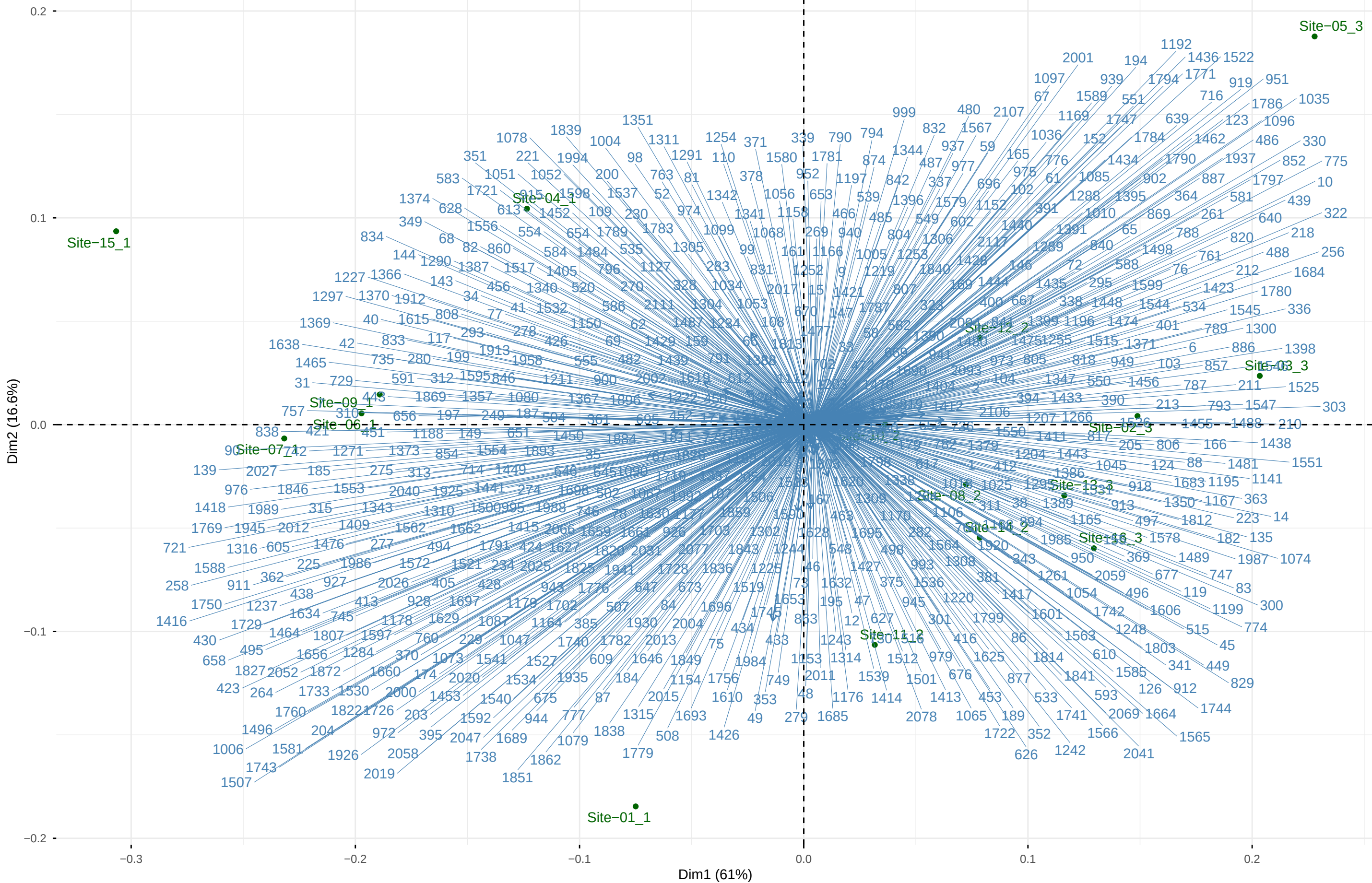
PCA – Biplot
