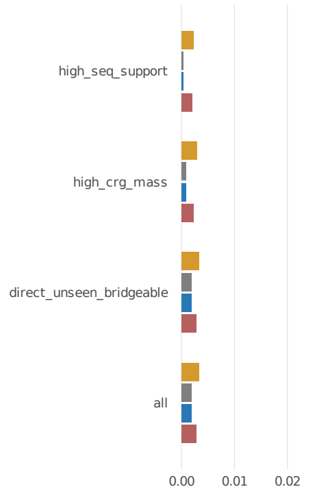
junyi
