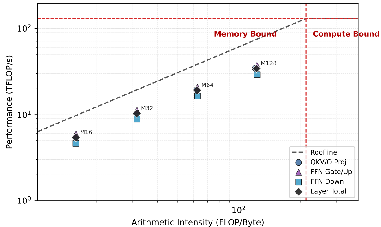
(b) LLaMA GEMM Roofline
