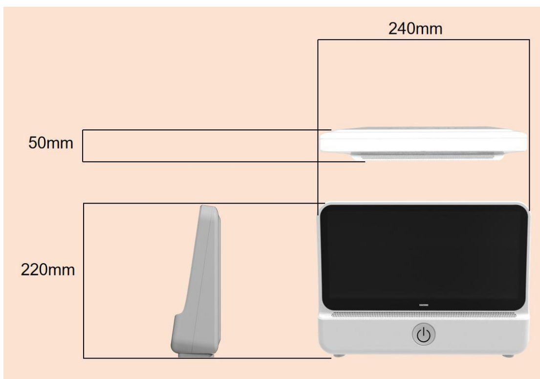
图 5-8 产品主体尺寸图（图片来源：作者自制）
