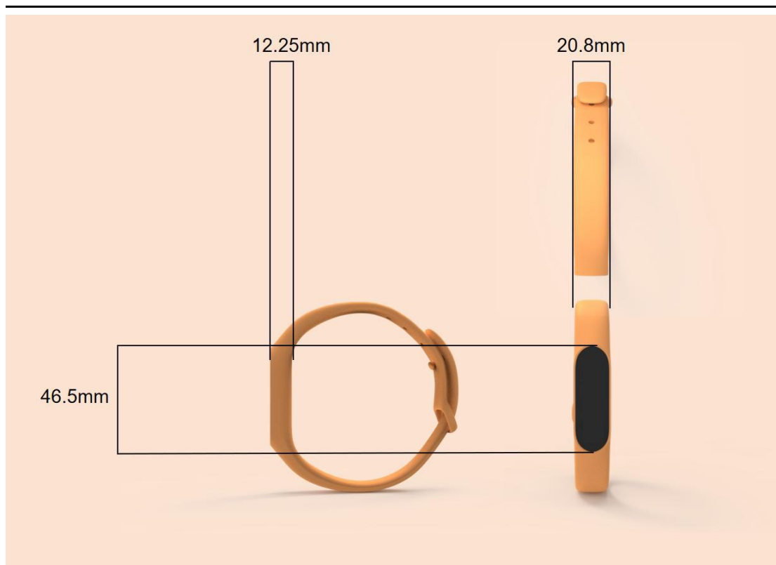
图 5-9 健康手环尺寸图（图片来源：作者自制）
