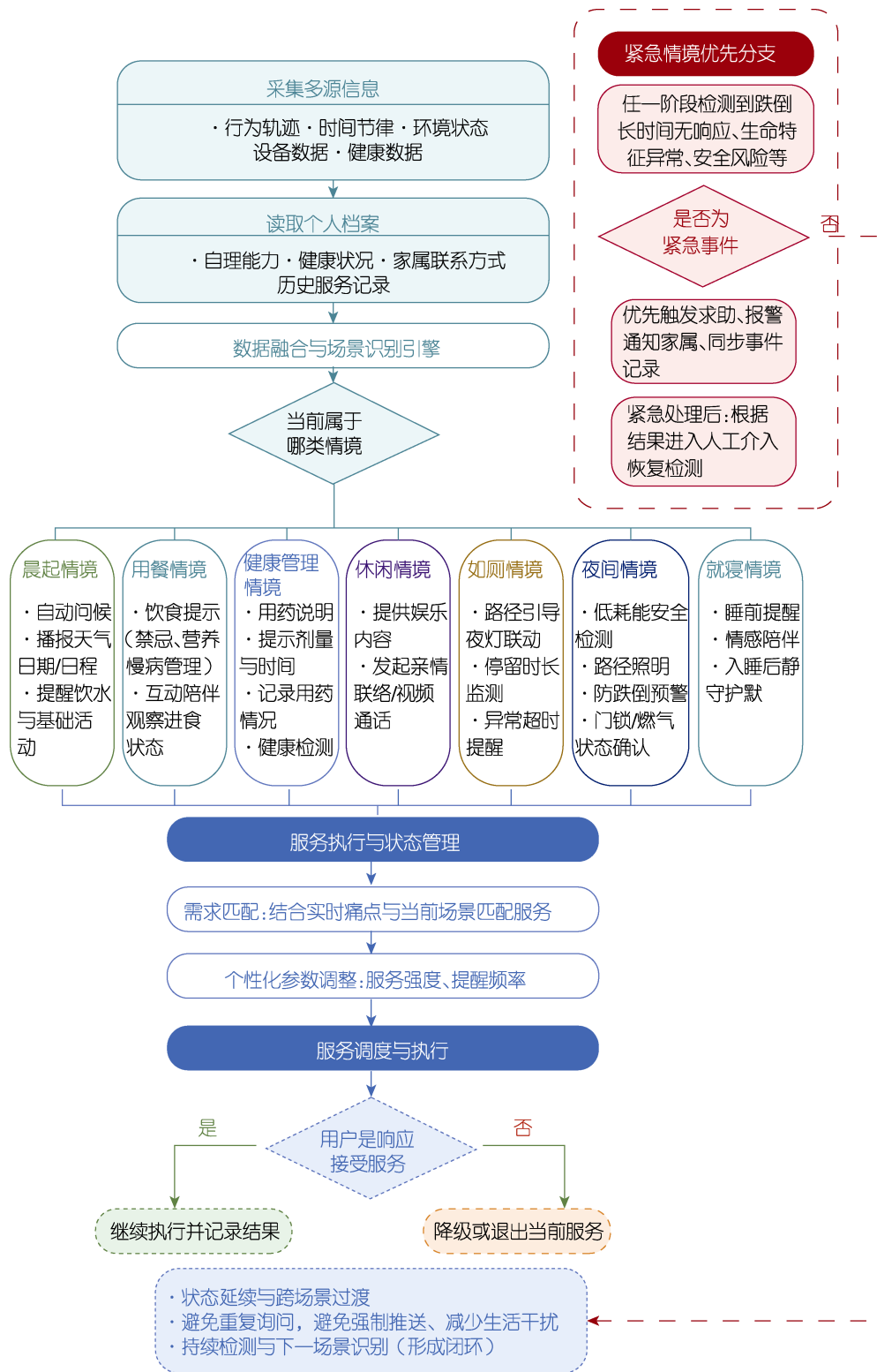
图 7 情境自适应的服务流程图 Fig.7 Flow chart of context-adaptive service
