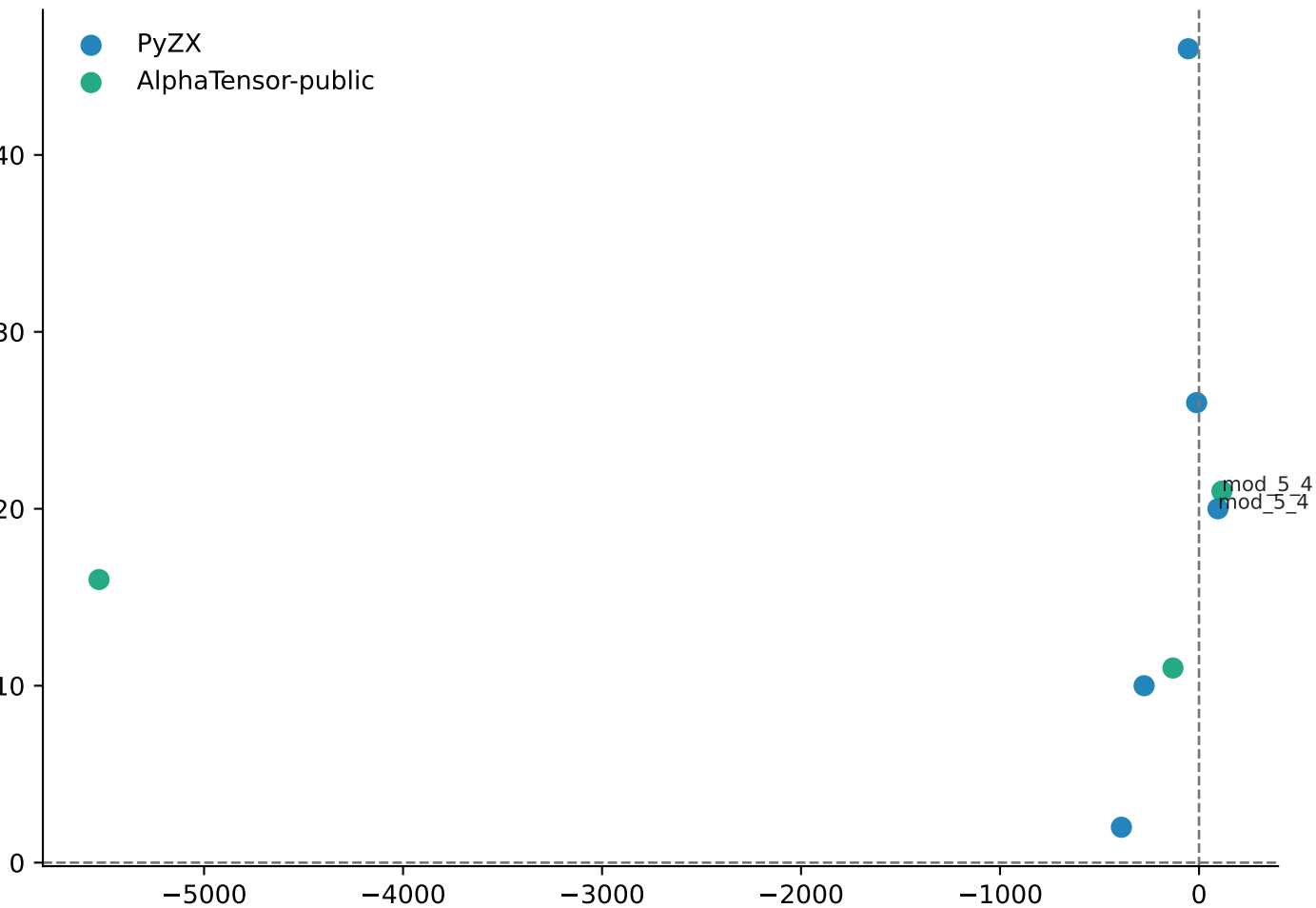
Reducao de T-count vs mudanca estrutural
