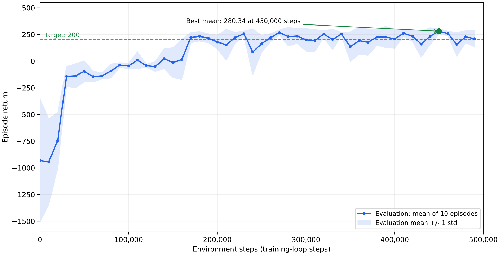
LunarLander-v2 | Double DQN | seed 1
